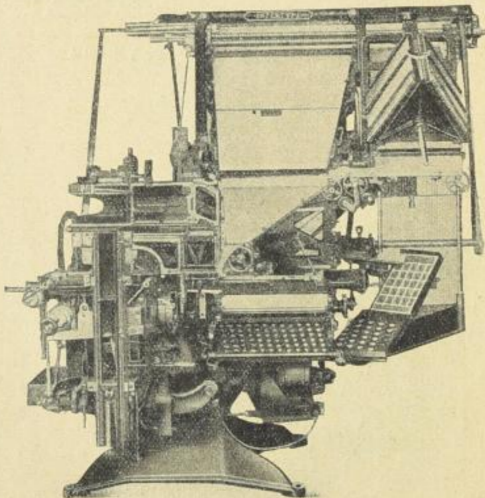
Die Intertype, erbaut unter Benutzung von Patenten der Linotype in Amerika. Dieses Modell hat drei Haupt- und drei Nebenmagazine
