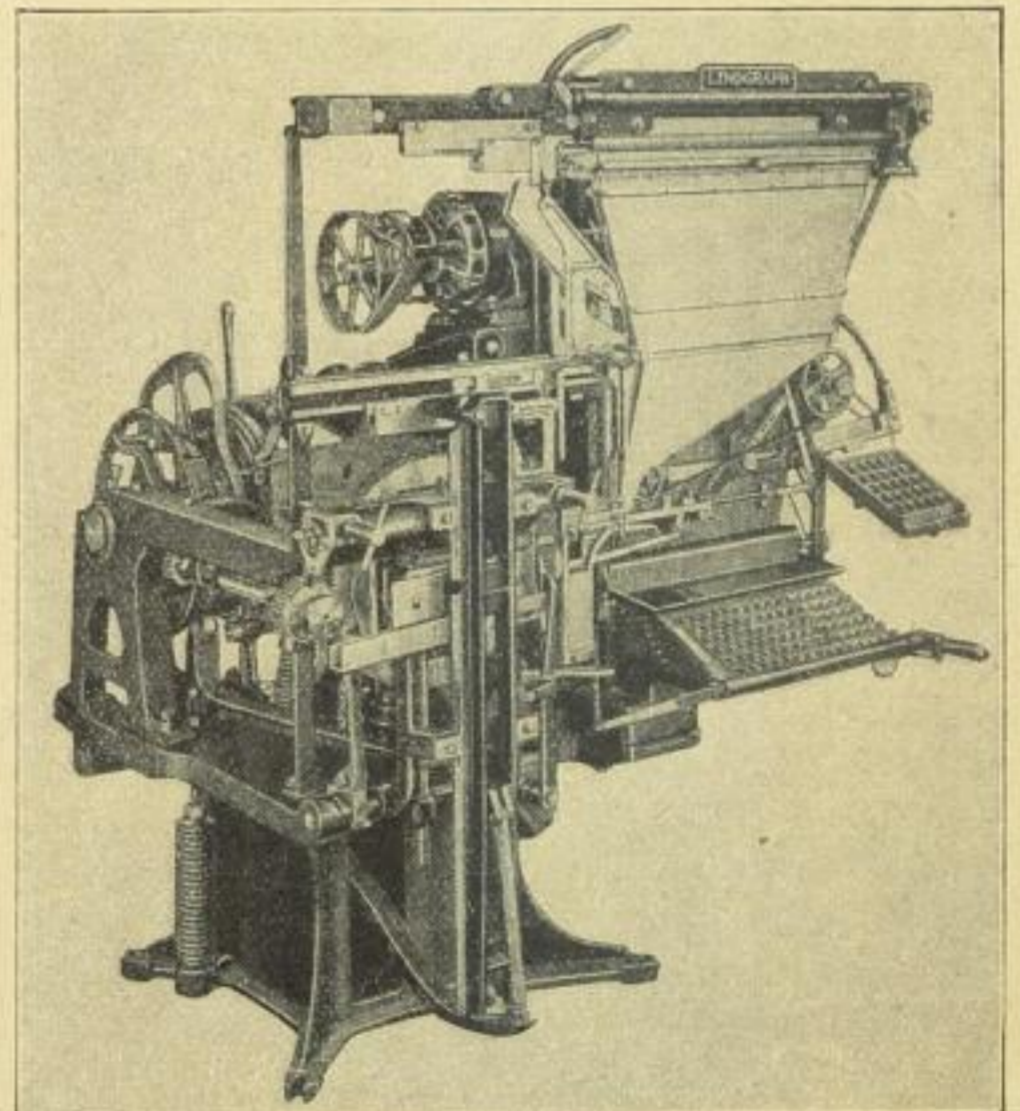
Die Linograph-Setzmaschine in Deutschland die „Darmstädter“ genannt; wird gebaut von der Firma Goebel in Darmstadt
