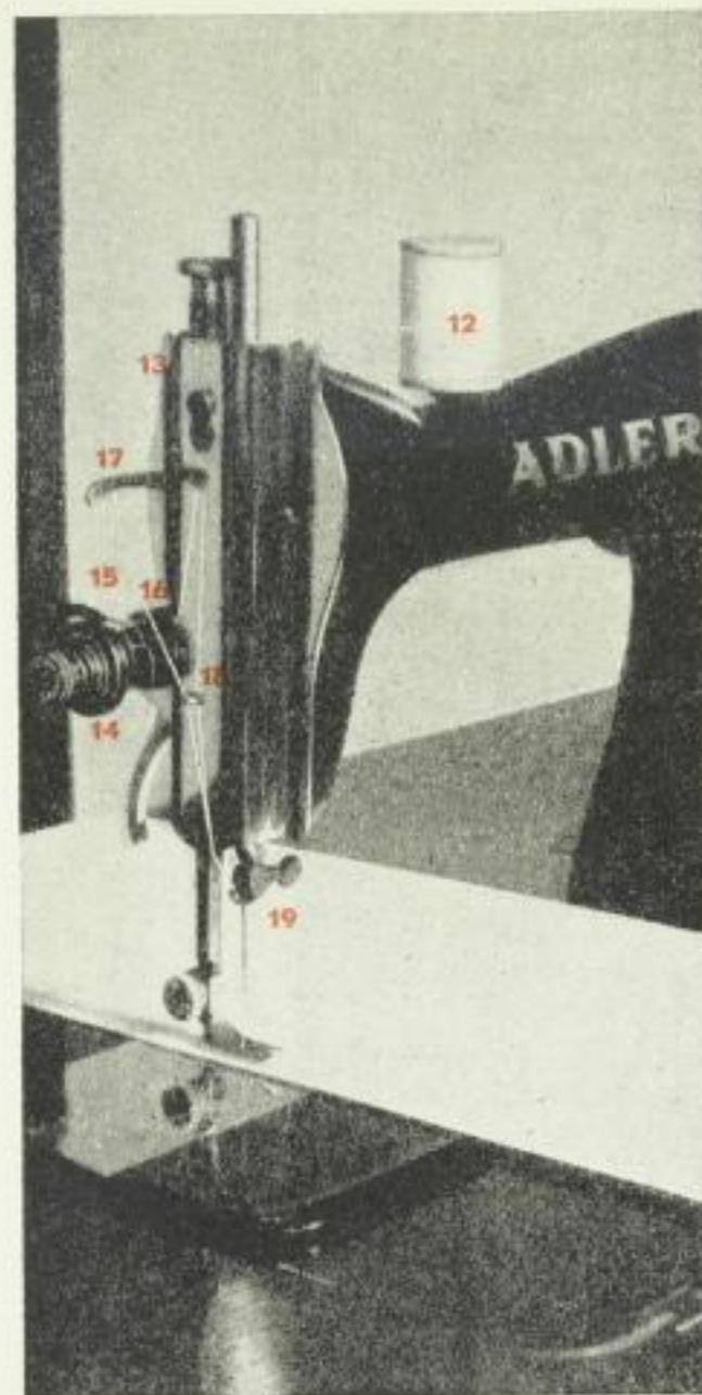
Fig. 5 Das Einfädeln des Nadelfadens
