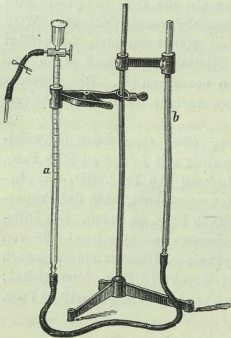
Fig. 1. Lunge'sches Nitrometer.
