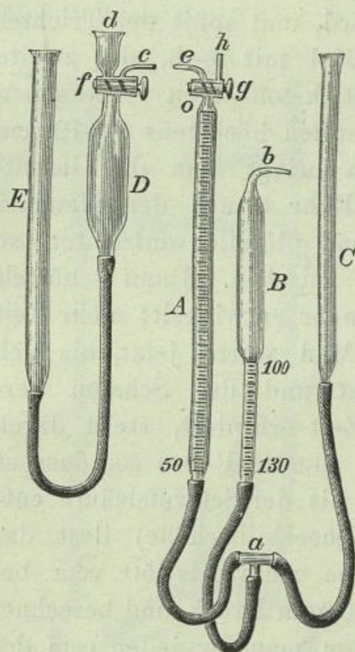
Fig. 2. Lunge'sches Gasvolumeter.
