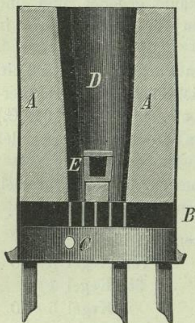
Fig. 5. Deville'scher Gebläseofen.
