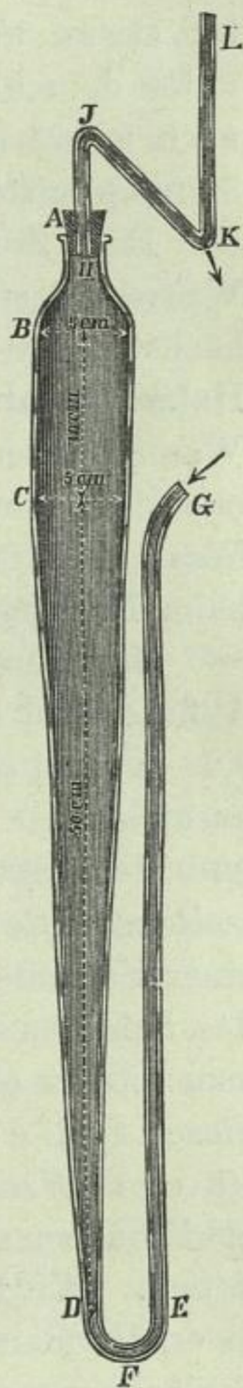
Fig. 4. Schlammapparat von Schöne.
