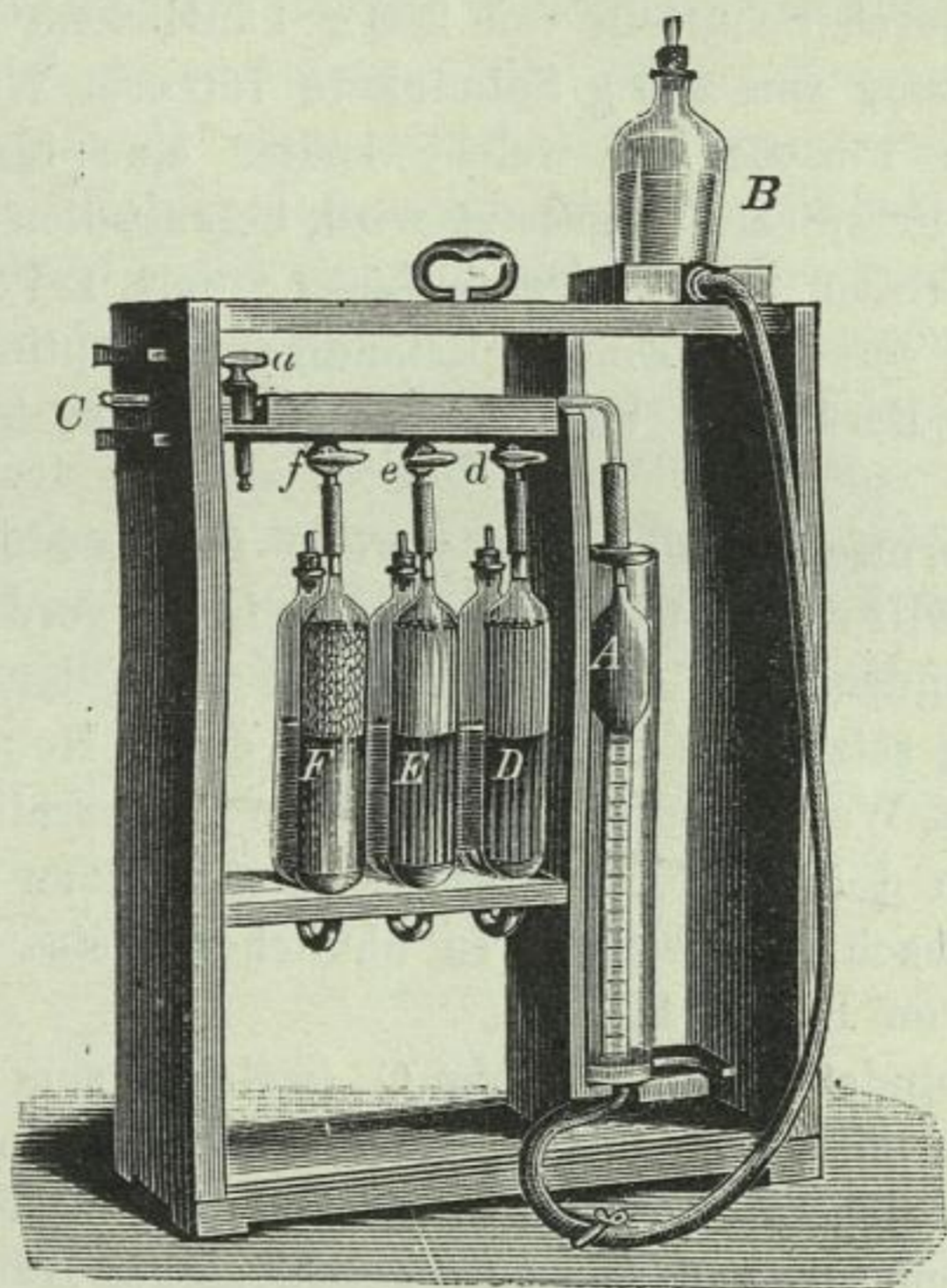
Fig. 3. Orsat'scher Apparat.
