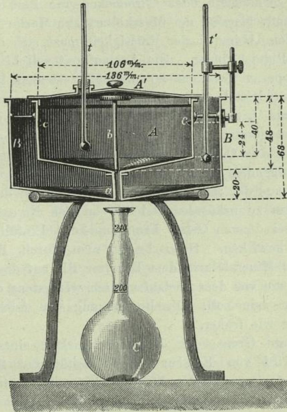
Fig. 11. Viscosimeter von Engler.
