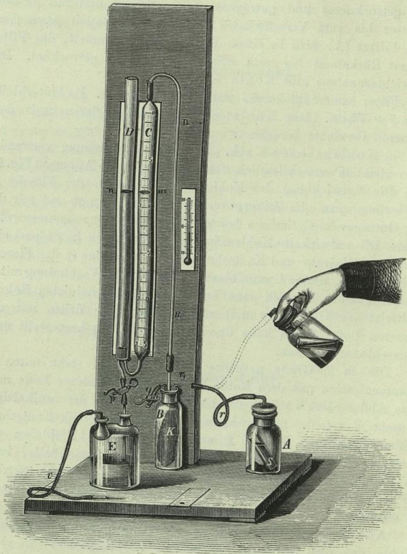
Fig. 9. Scheibler'scher Apparat.
