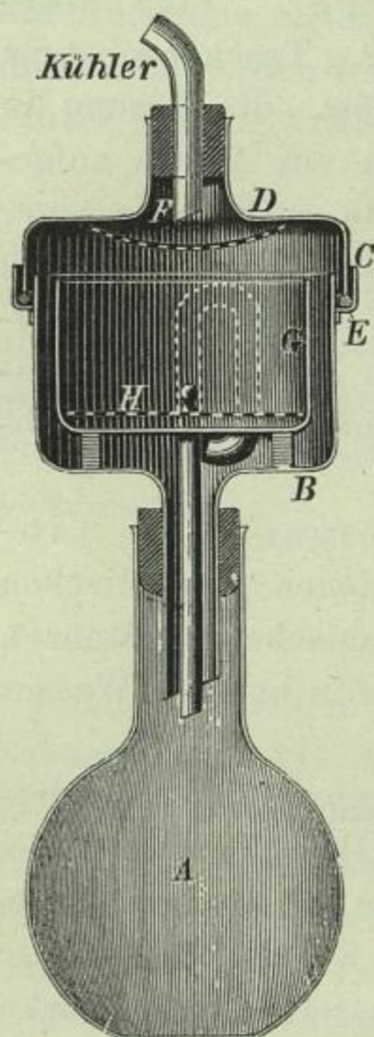
Fig. 11. Extractions-Apparat für Gerbmaterien.
