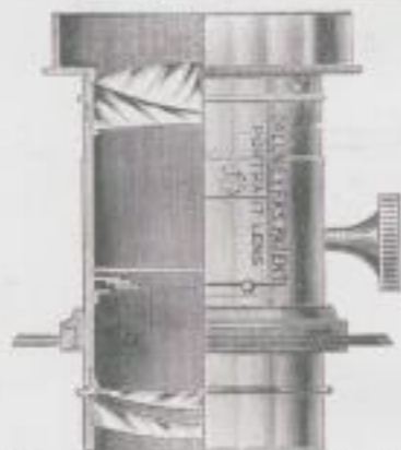
Patent-Portr.-Obj. Serie B. Dallmeyer, London.
