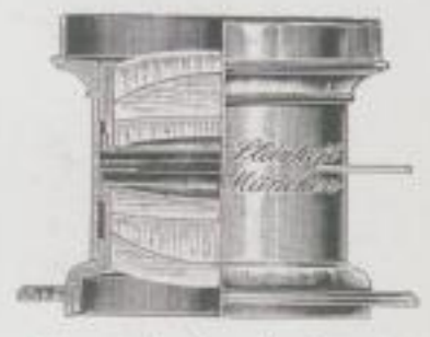
Reproductions-Aplanat. C. A. Steinheil Söhne, München.
