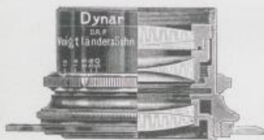
Dynar. Voigtländer & Sohn, Braunschweig.
