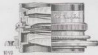
Tessar. Carl Zeiß, Jena.
