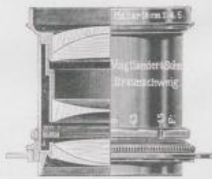
Heliar. Voigtländer & Sohn, Braunschweig.
