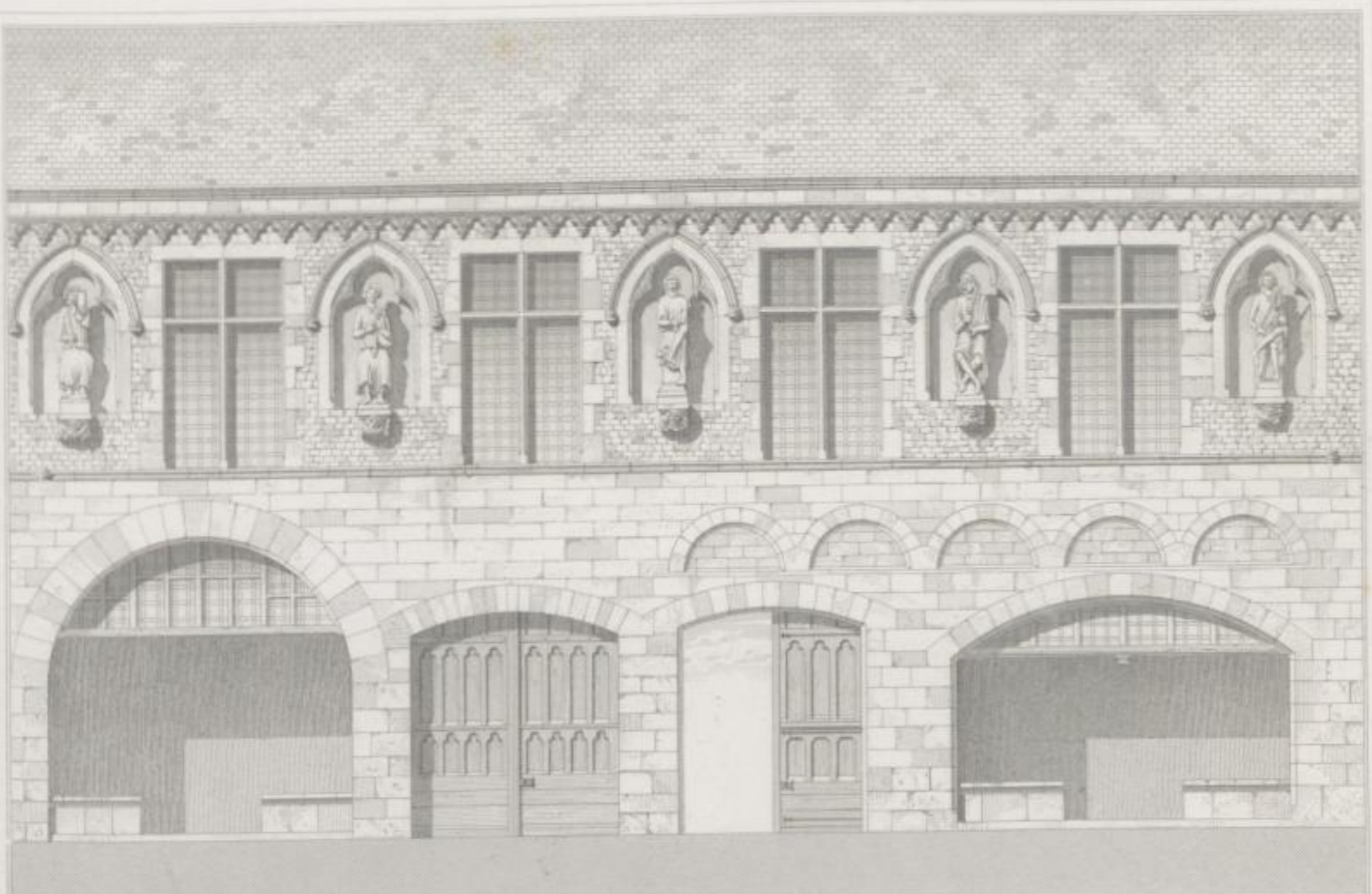
Elevation à 0, 005 p. mètre.
