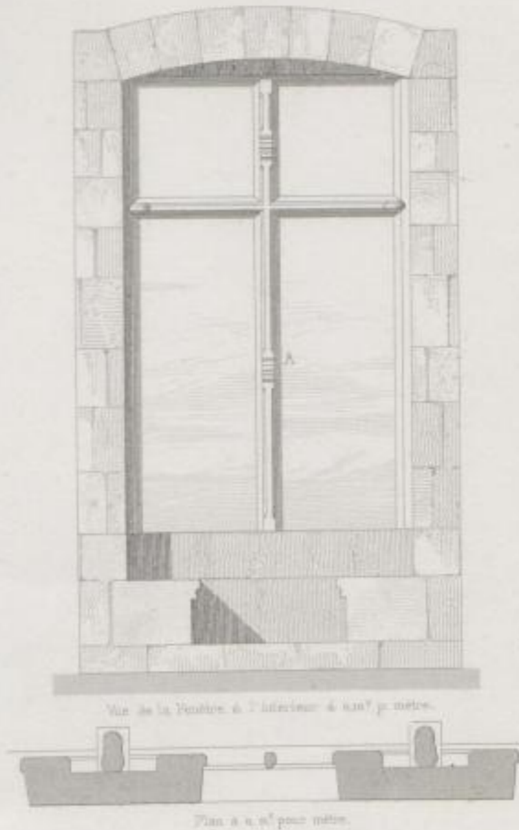
Plan à 0,01 p. mètre.
