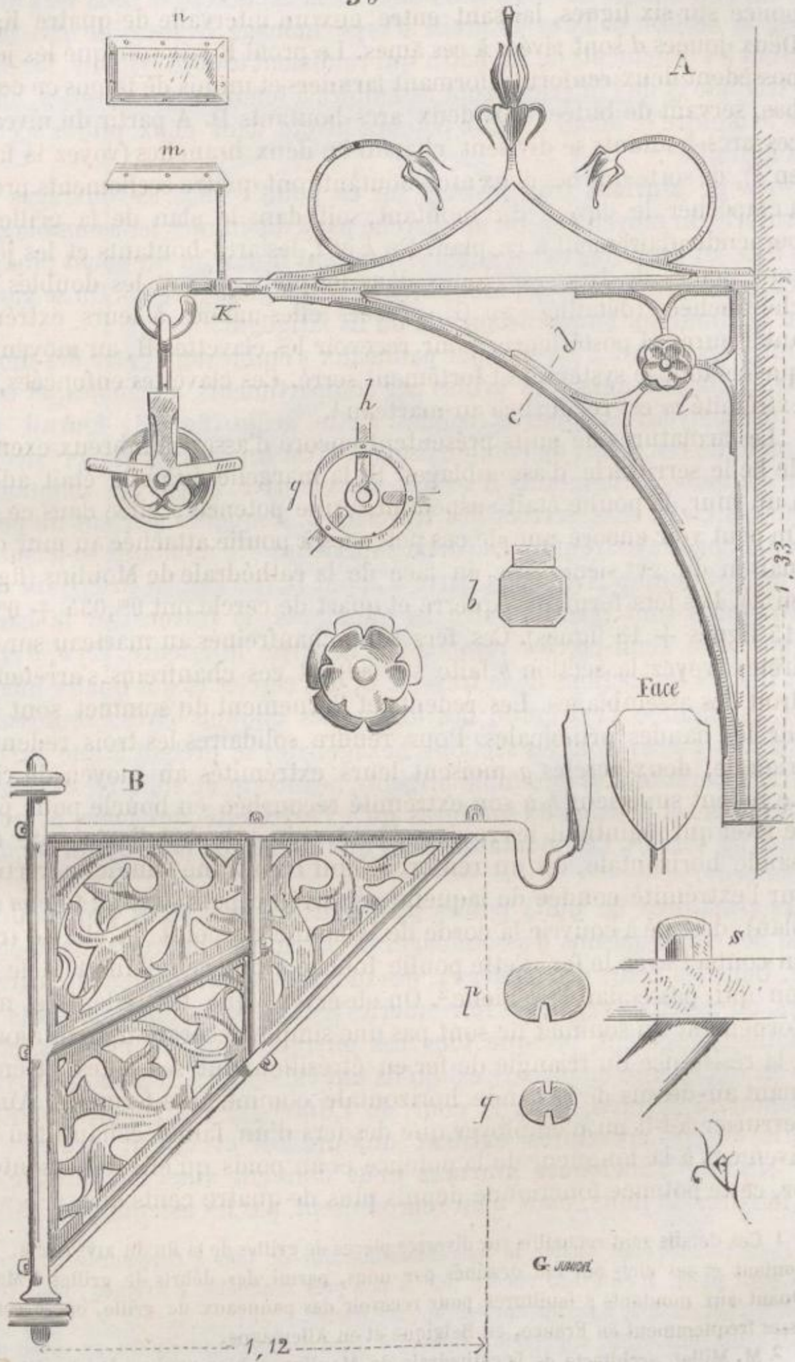
En B, est figurée une seconde potence, composée d'après un autre
