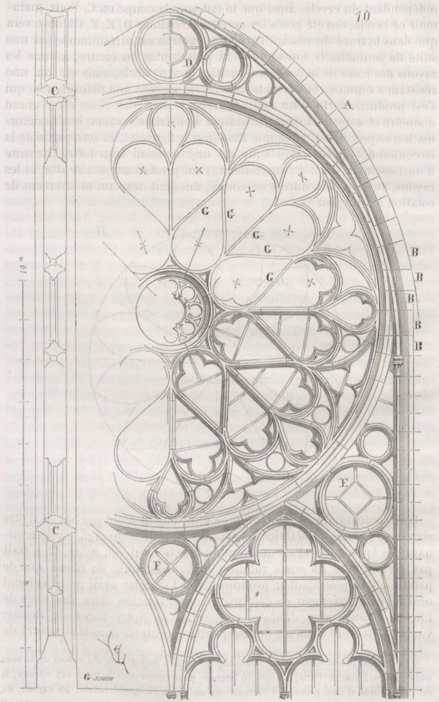
cinq sommiers B. Le réseau est, conformément à la donnée rémoise,
