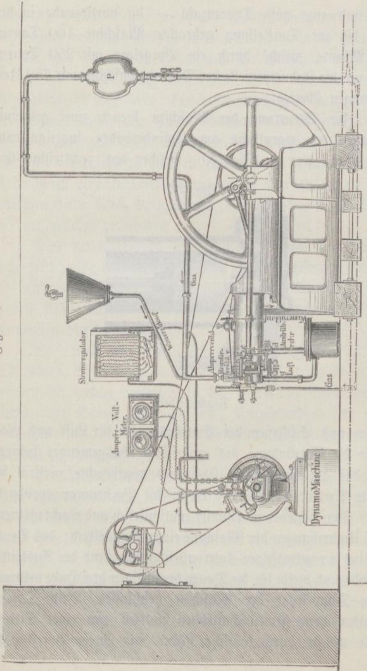
Verbindung des Motors mit der Dynamo.
