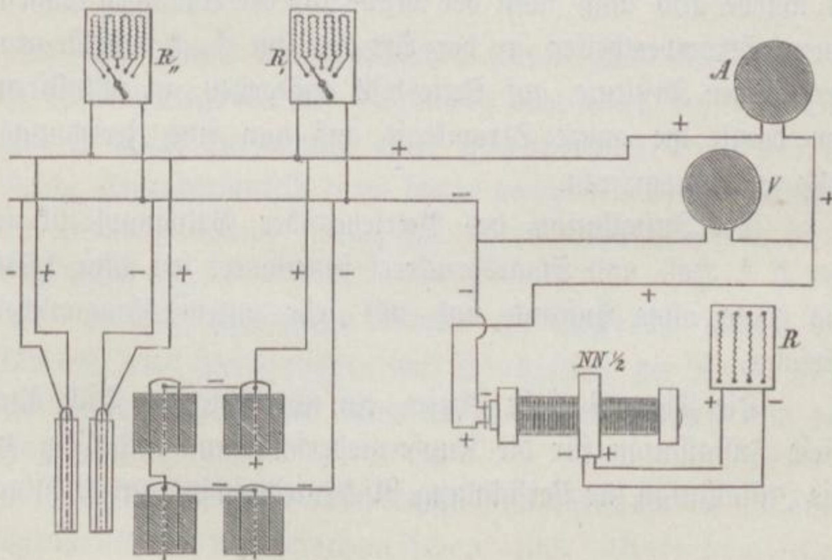
Bäder für Verstählung und Vernickelung.
