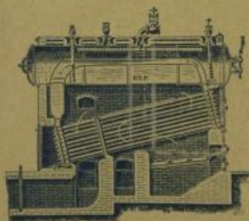
Büttner-Patent-Schnellumlaufoessel.
