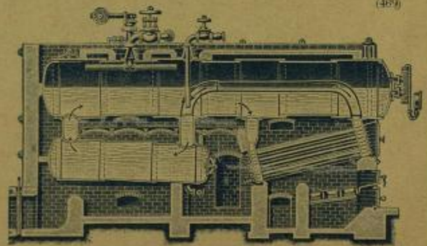
Büttner-Patent-Grosswasserraumkessel.
