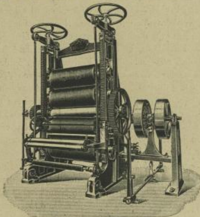
Calander mit 5 Walzen.
