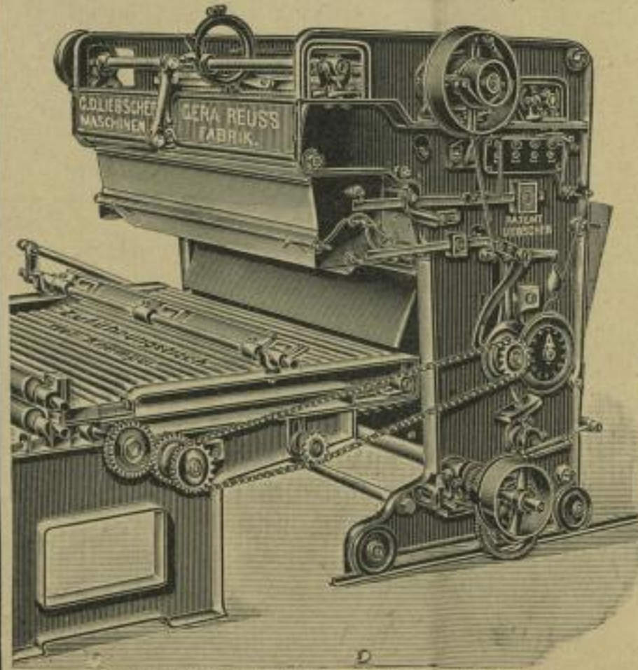
Speisemaschine für Baumwollabdruckempeln.
