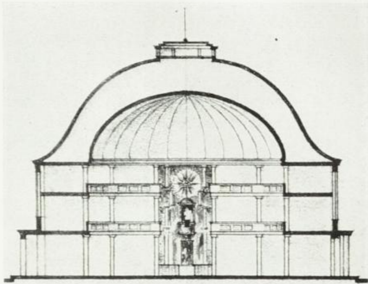
120. Krotoschin (Posen), Schnitt
