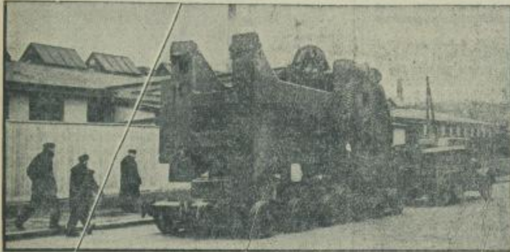
Die Vorbereitungen für die Leipziger Frühjahrsmesse 1939 sind in vollem Gange. — Eine hydraulische Schraubepresse für 800 Tonnen Pressdruck beim Transport auf dem Culemmer-Straßenfahrzeug zur Halle 11a für die Große Technische Messe und Baumesse in Leipzig, die in der Zeit vom 5. bis 13. März 1939 stattfindet. (Weltbild-Wagenborg - M.)
