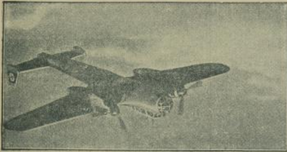
Das neue Kampfflugzeug Dornier Do. 215. Das Kampfflugzeug Dornier Do. 215 trägt die Tradition des bewährten Kampfflugzeuges Dornier Do. 17. Die Leistungen dieser Neukonstruktion konnten gegenüber der Do. 17 noch gesteigert werden. Neuartig auffällig ist bei diesem zweimotorigen Ganzmetall-Eindecker der überaus markante planvergente noch vor der Schraubenebene liegende Kopf, der einer aus vier Mann bestehenden Besatzung in idealster Weise für Flug und Kampf Raum bietet. (Bild: Wagners — M.)
