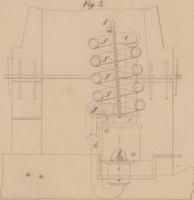
Hauptstube für das Frischfeuer zu Hausen.
