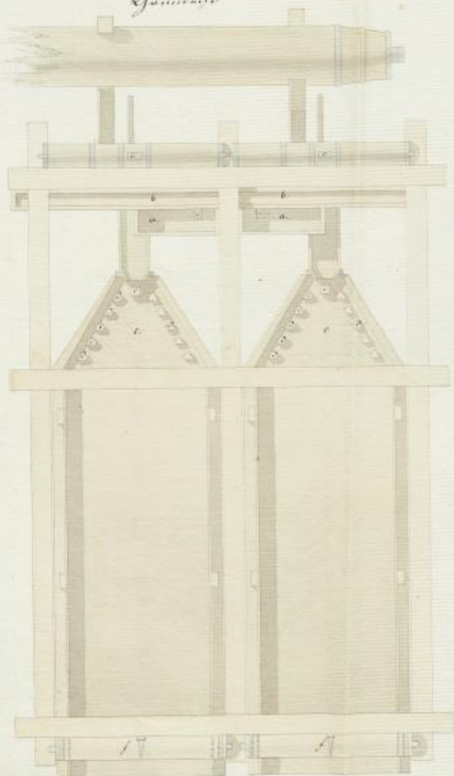
Grundriß
