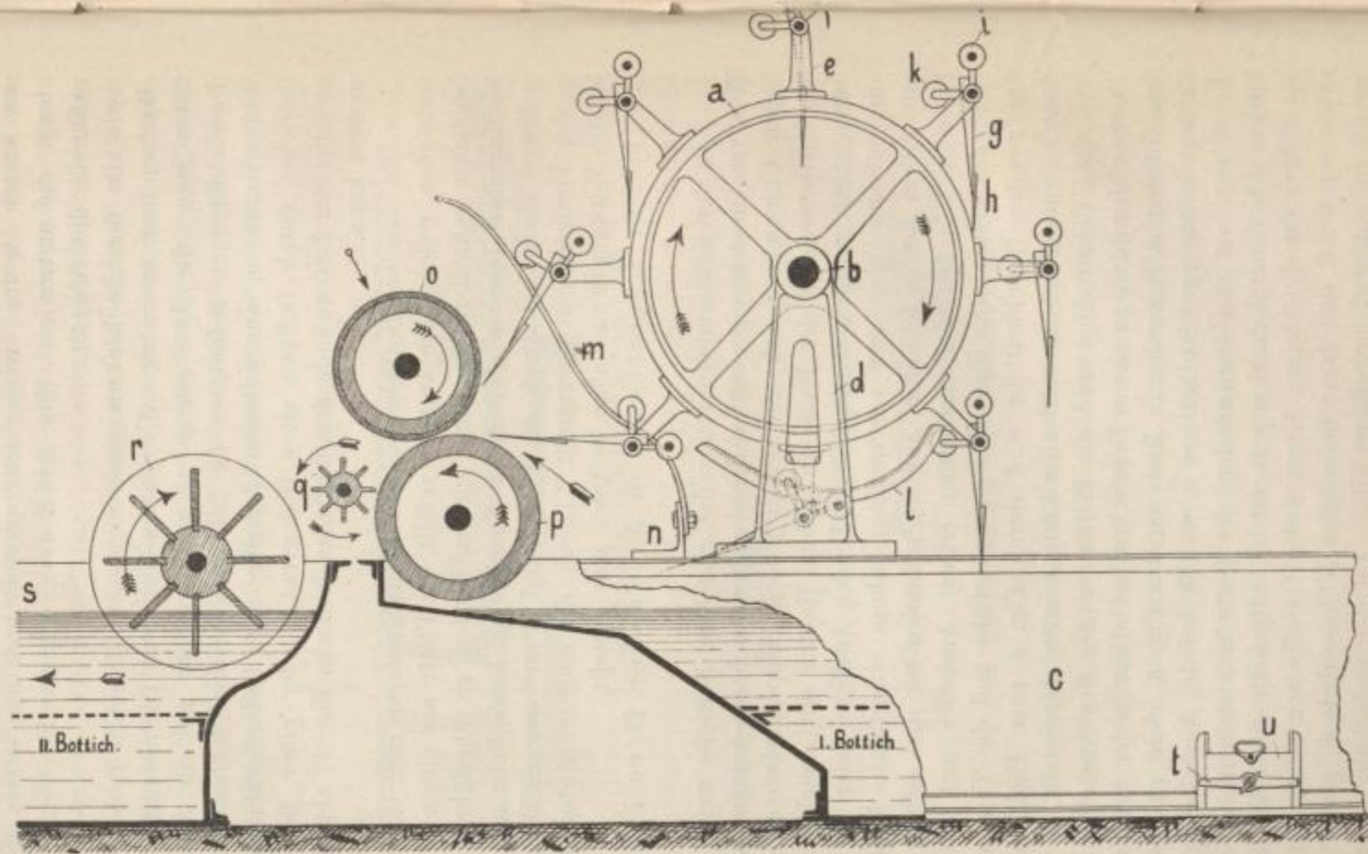
Fig. 4. Der Leviathan von Alexander Déru. (Verticalsechnitt).
