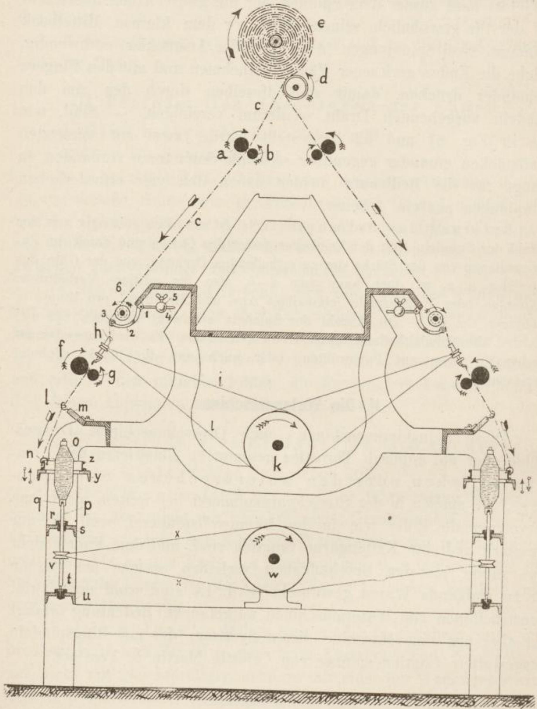
Fig. 67. Der Continuespinner von Martin. (Verticalschnitt.)
