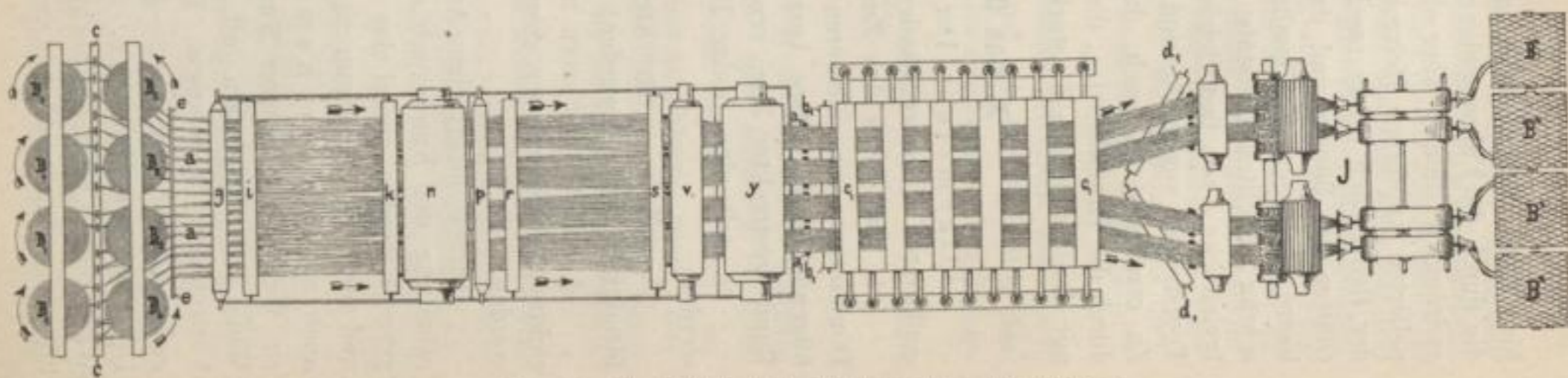
Fig. 85. Die Köchlin'sche Plättmaschine. (Draufsicht.)
