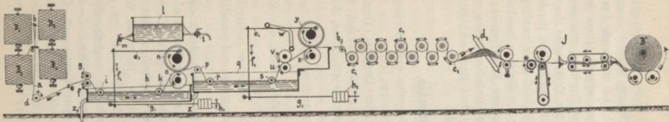
Fig. 84. Die Köchlin'sche Plättmaschine. (Verticaler Längenschnitt.)
