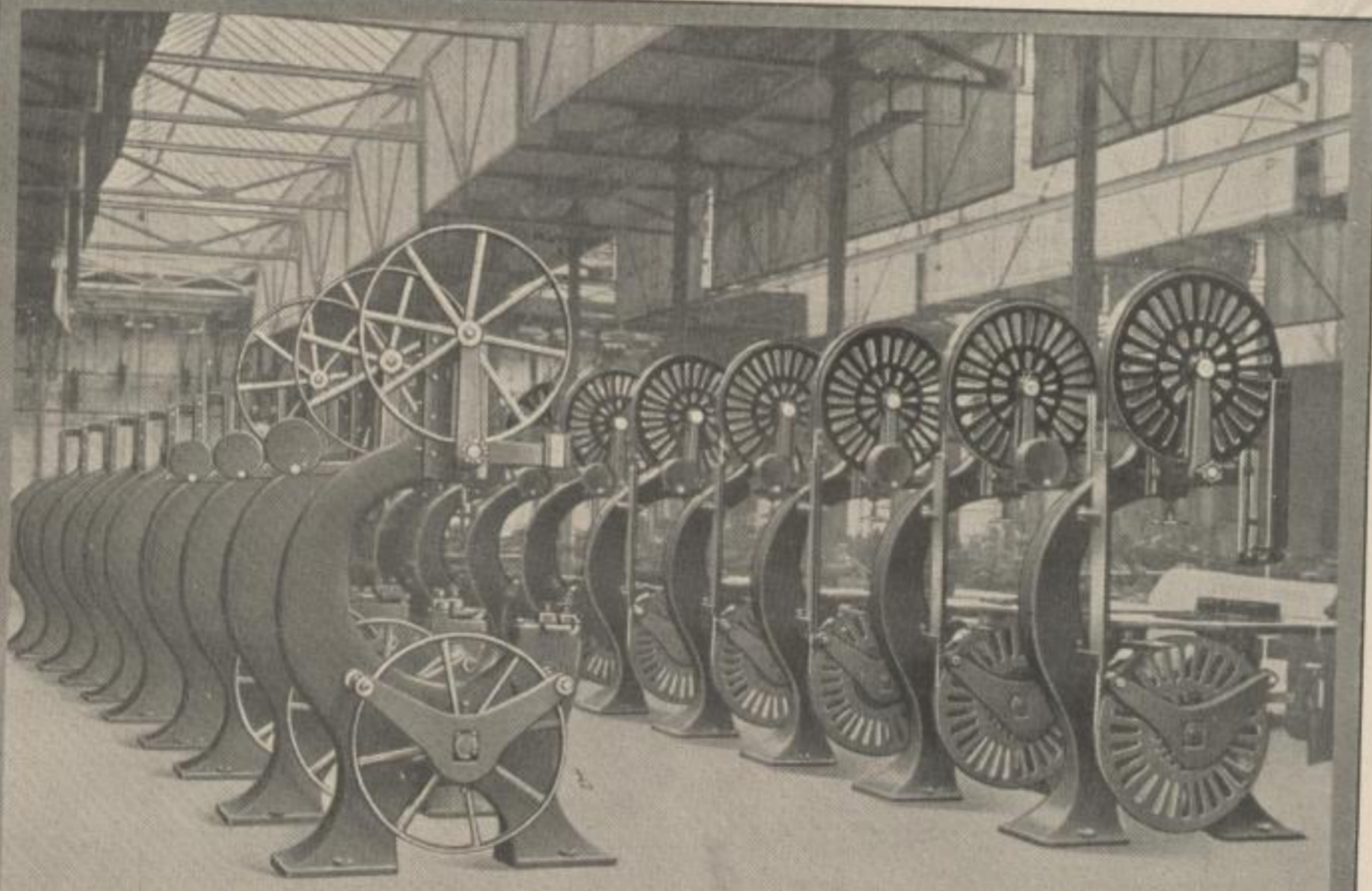
Montage I Bandsägen.
