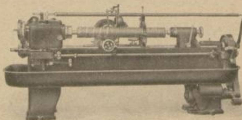
Universal-Gewindefräsmaschine Modell B 2 E mit Einscheiben- und elektr. Antrieb
