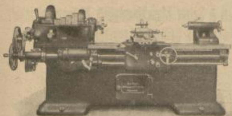
Universal-Hinterdrehbank Modell UH D 5 L mit Leitspindel und Schaftwelle
