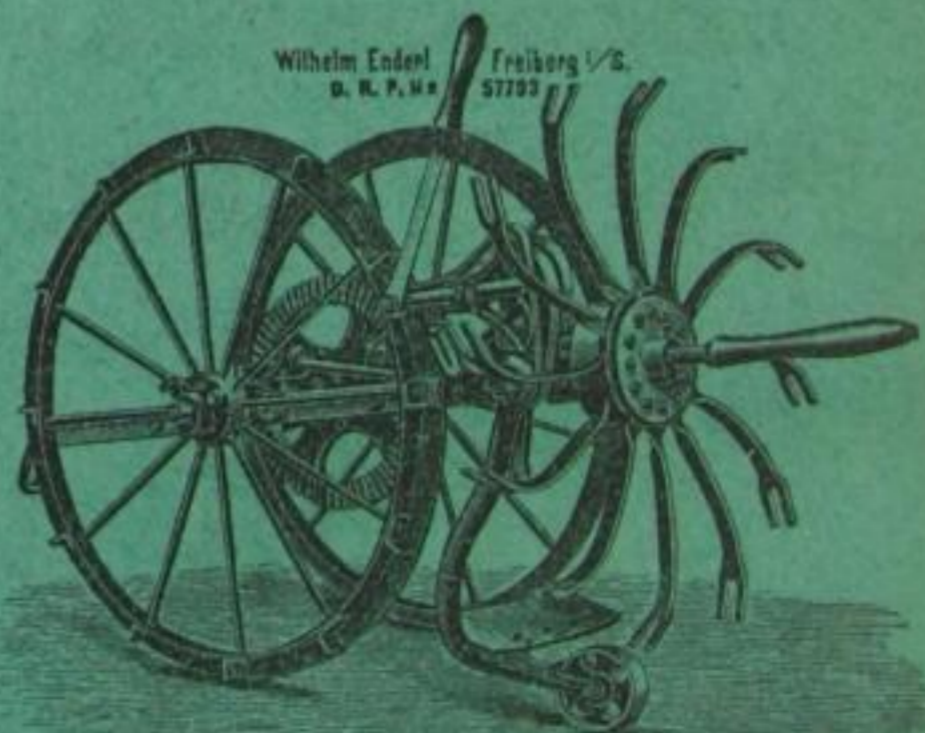
Kartoffelerntemaschine.
