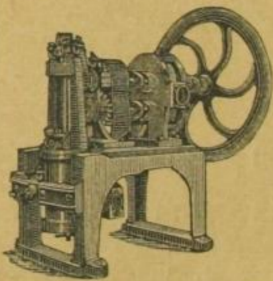
Rotirende Pumpe zu directem Dampftrieb, von 100—5000 Liter pro Minute liefernd.
