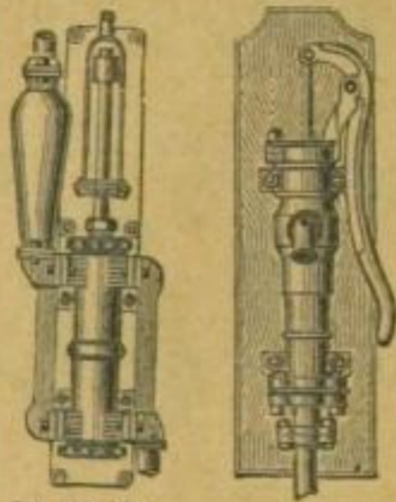
Doppeltw. Saug- und Druckpumpe ohne Antrieb.
