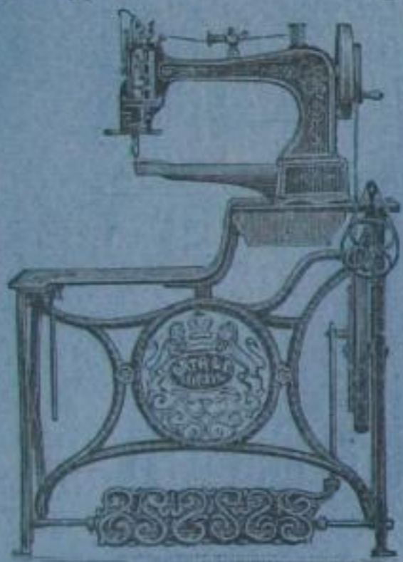
Original-Pallas-Elastik Neueste Schuhm.-Nähmaschine mit Rundtransporteur.
