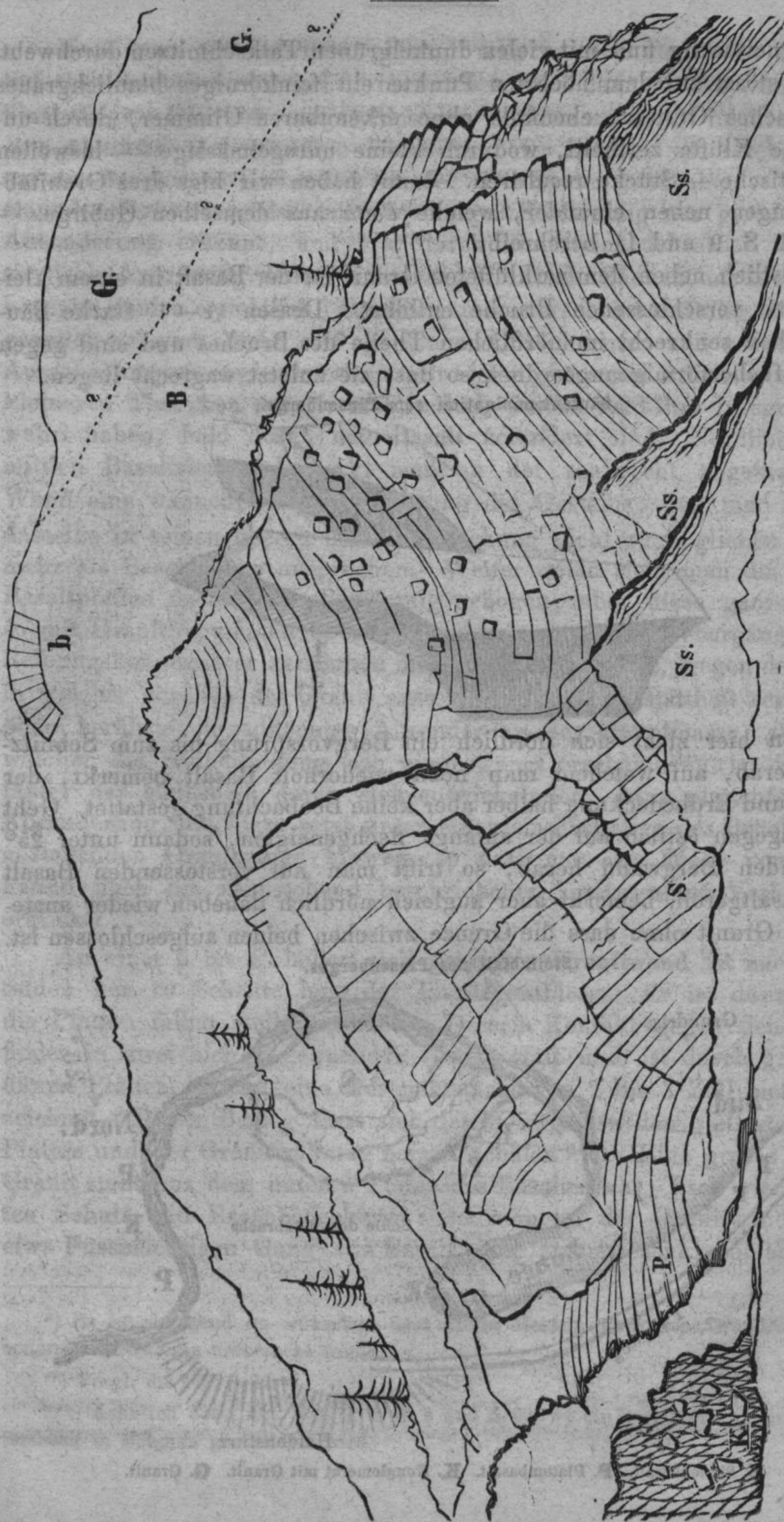
Basaltbruch auf der Ostseite des Pilsenberges skizzirt von A. von Gutbier 1856.
