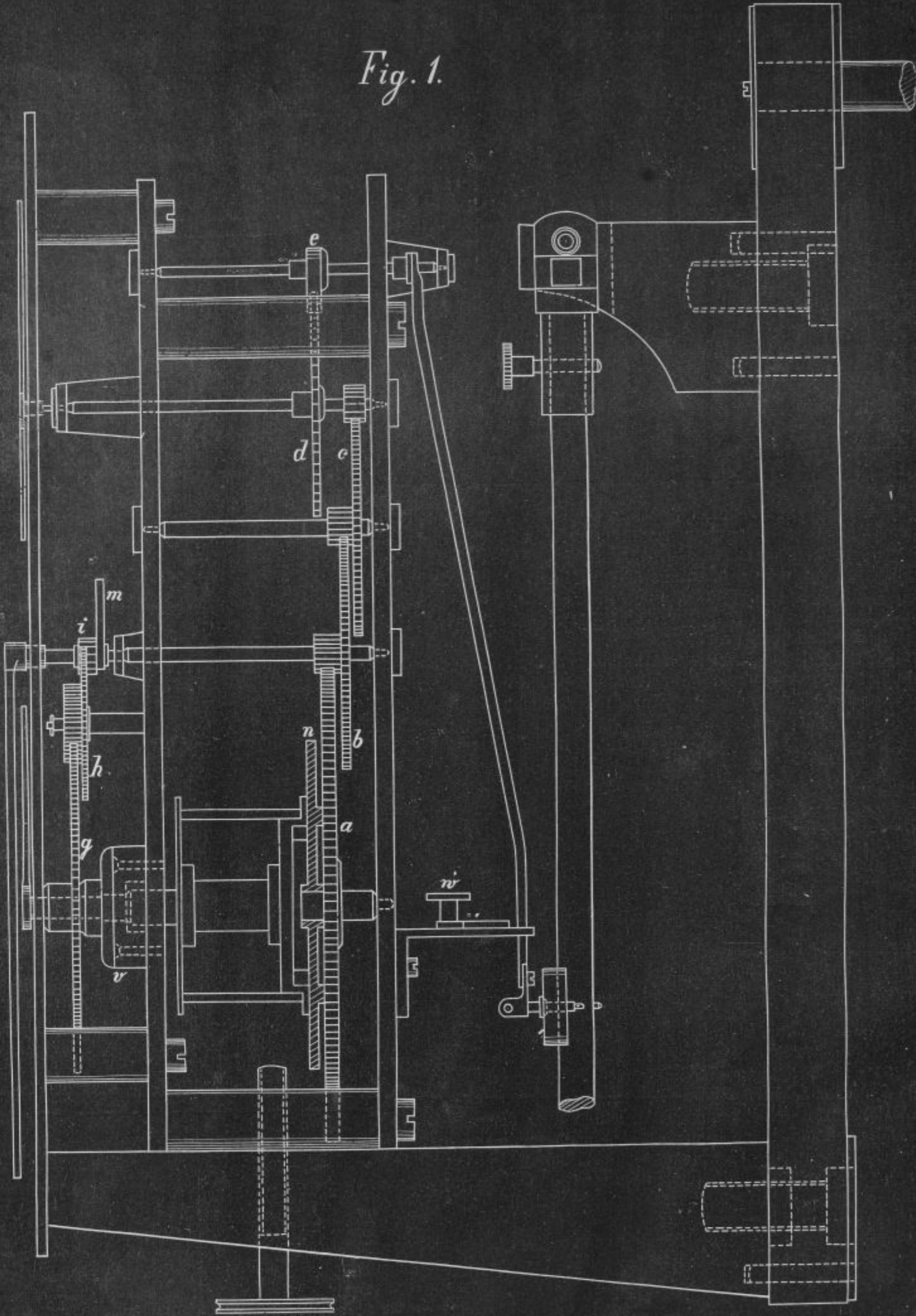
Seitenansicht einer astronomischen Pendeluhr.
