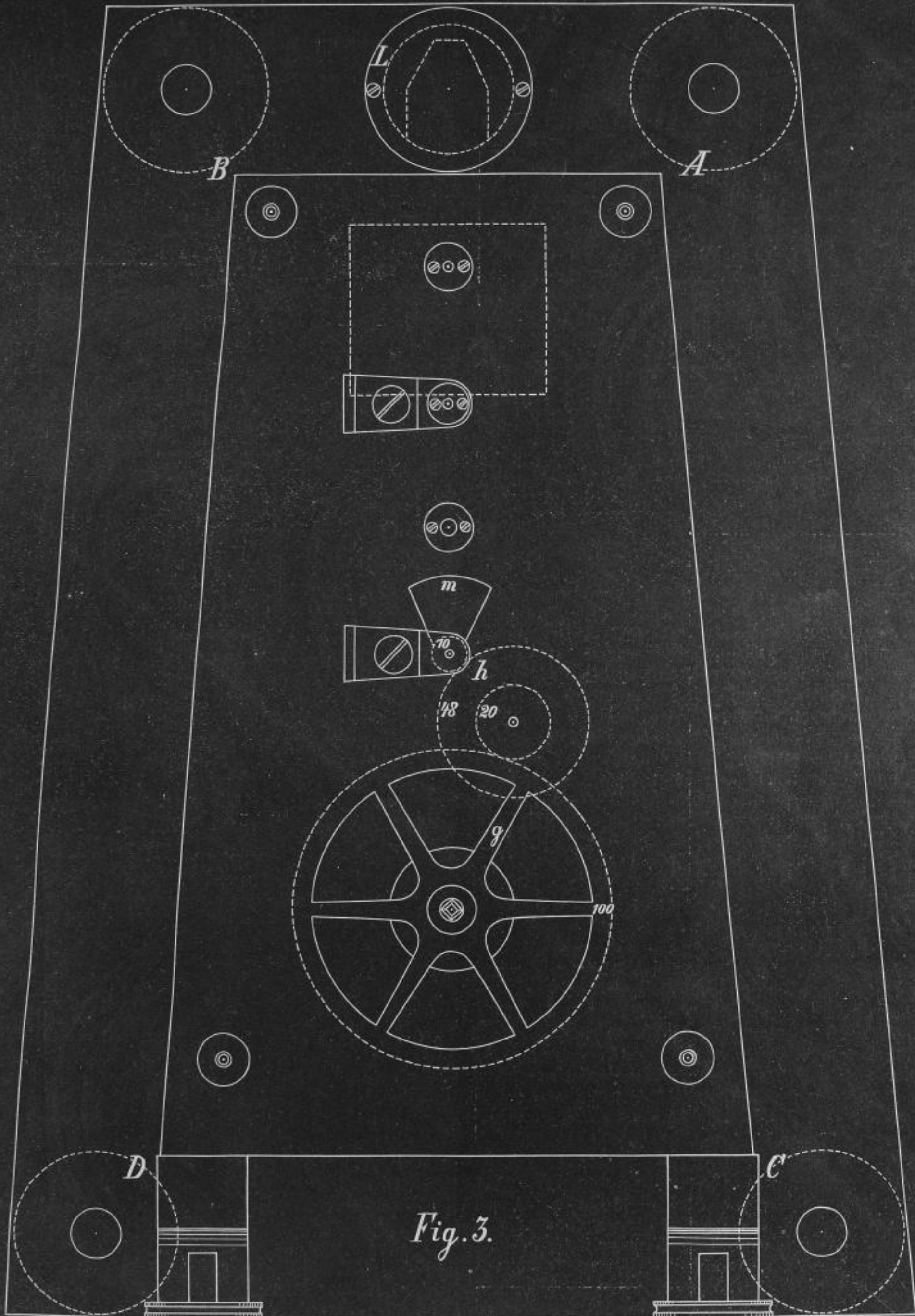
Gehört zu dem Artikel: „Ueber die Anfertigung einer astronomischen Pendeluhr“ von G. Ph. Völling (Siehe Nr. 5, S. 69, Anmerkung)
