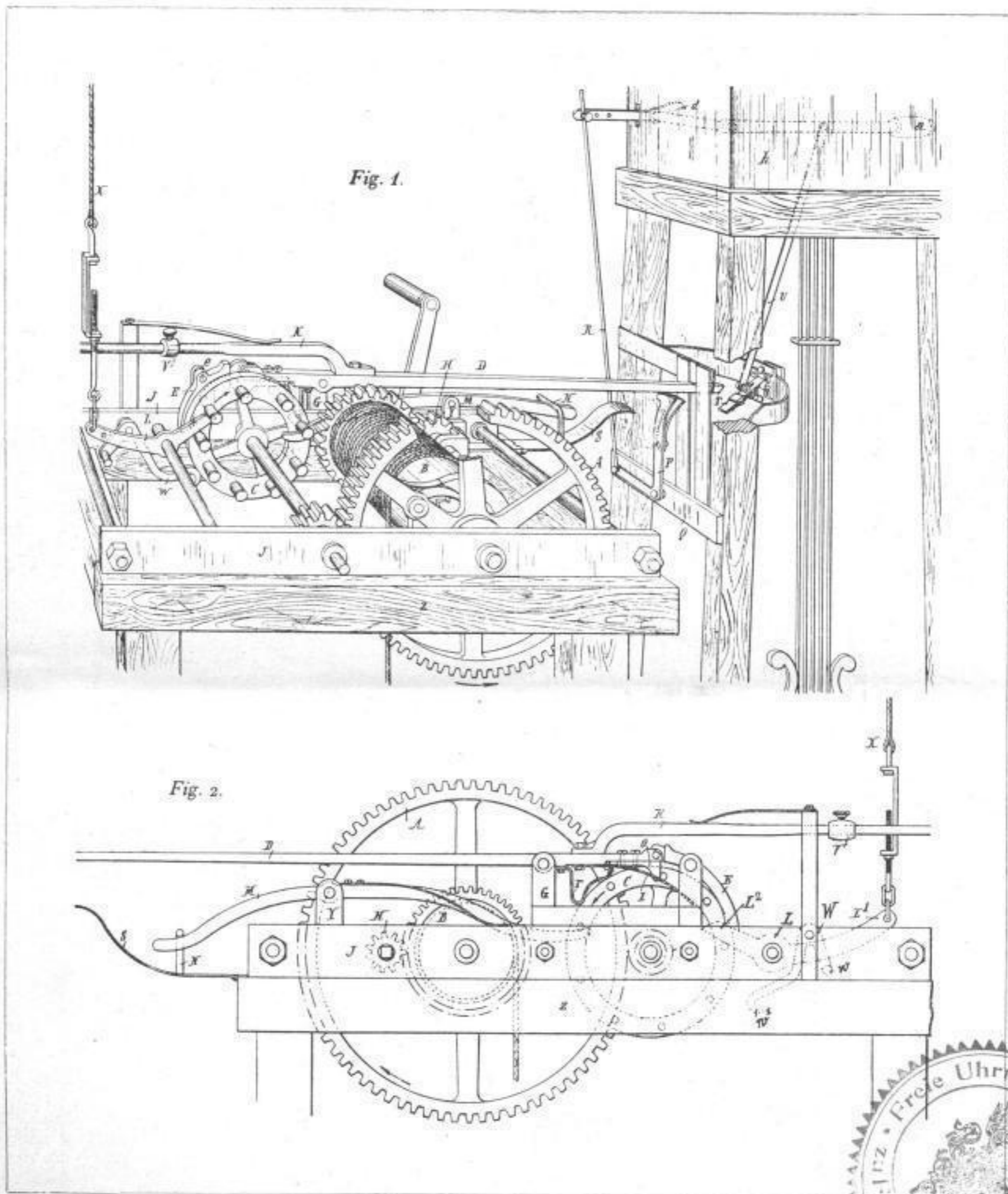
Schlagwerk für Turmuhren, von Valentin Jean-Marie in Bruyères (Frankreich).
