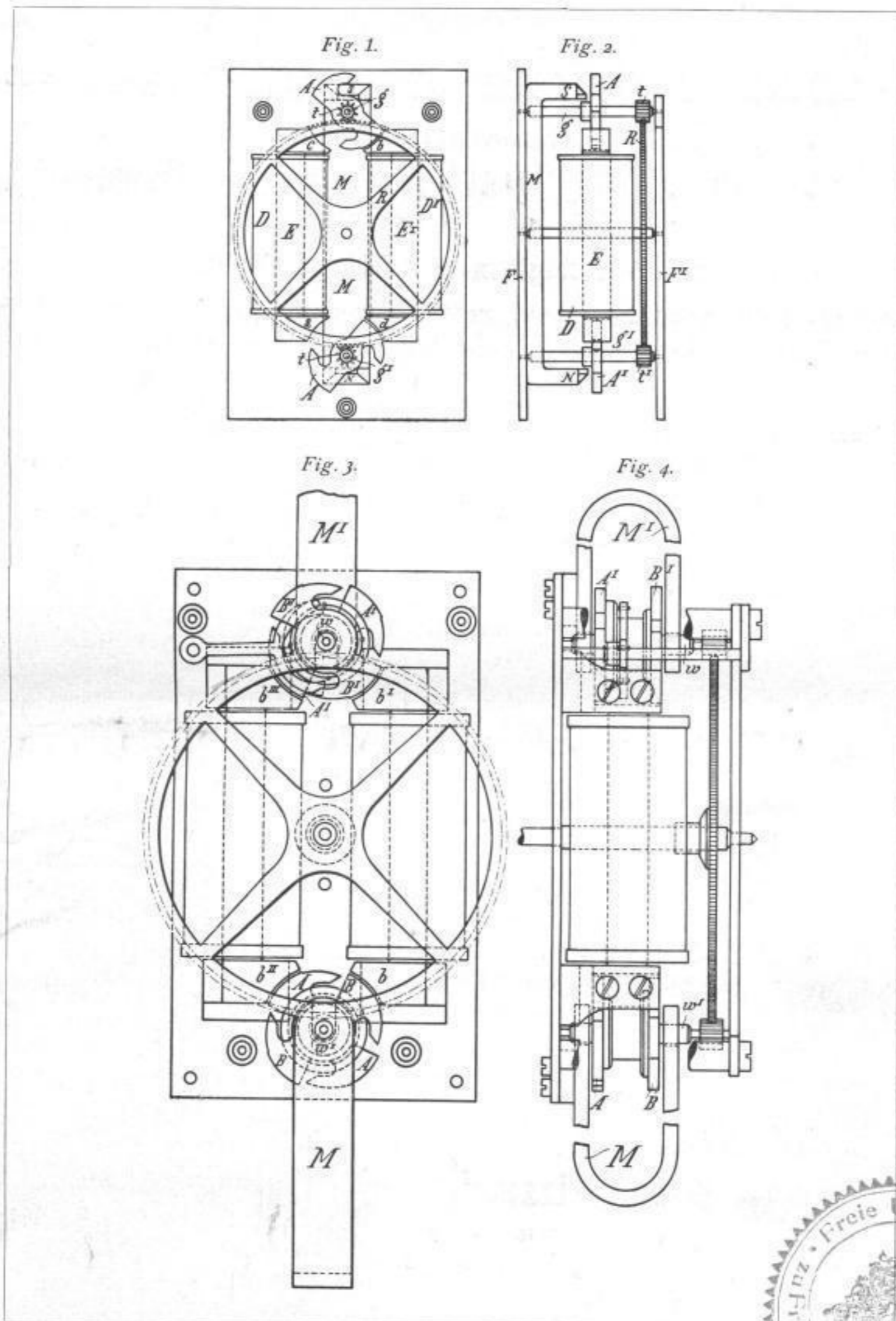
Wechselstrom-Nebenuhr, von H. Ch. Spohr in Frankfurt a. M.
