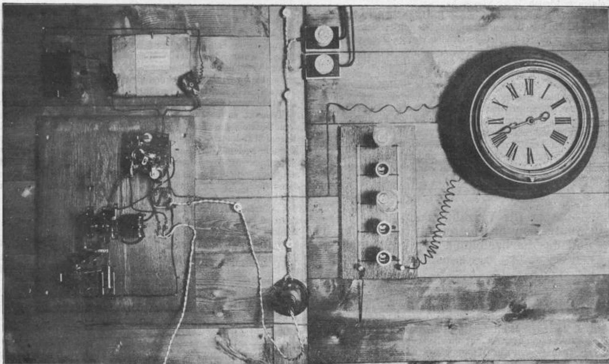
Inneres der Empfangsstation in Breitensee. Chronometrischer Apparat zur Verhütung von Störungen durch fremde Wellen oder atmosphärische Entladungen.
