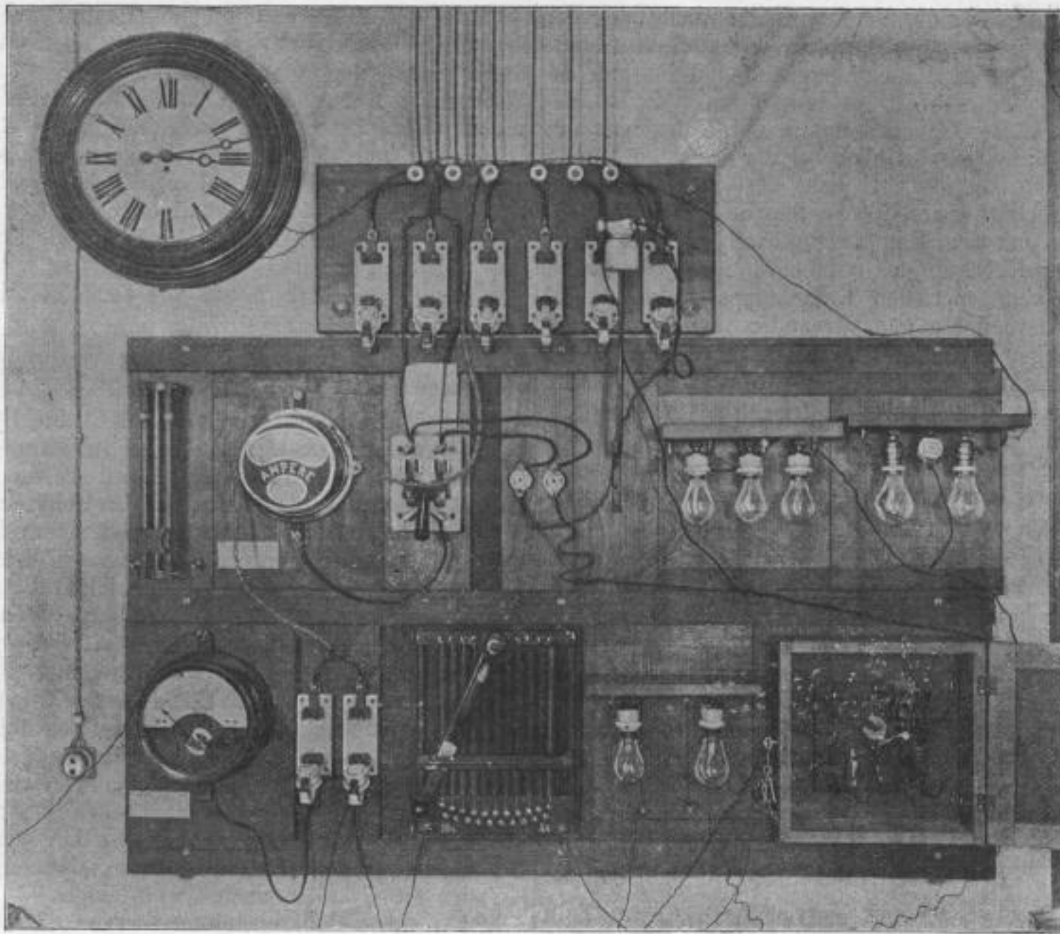
Inneres der Zentralstation. Das Schaltbrett mit den Hochspannungs-Schaltapparaten.
