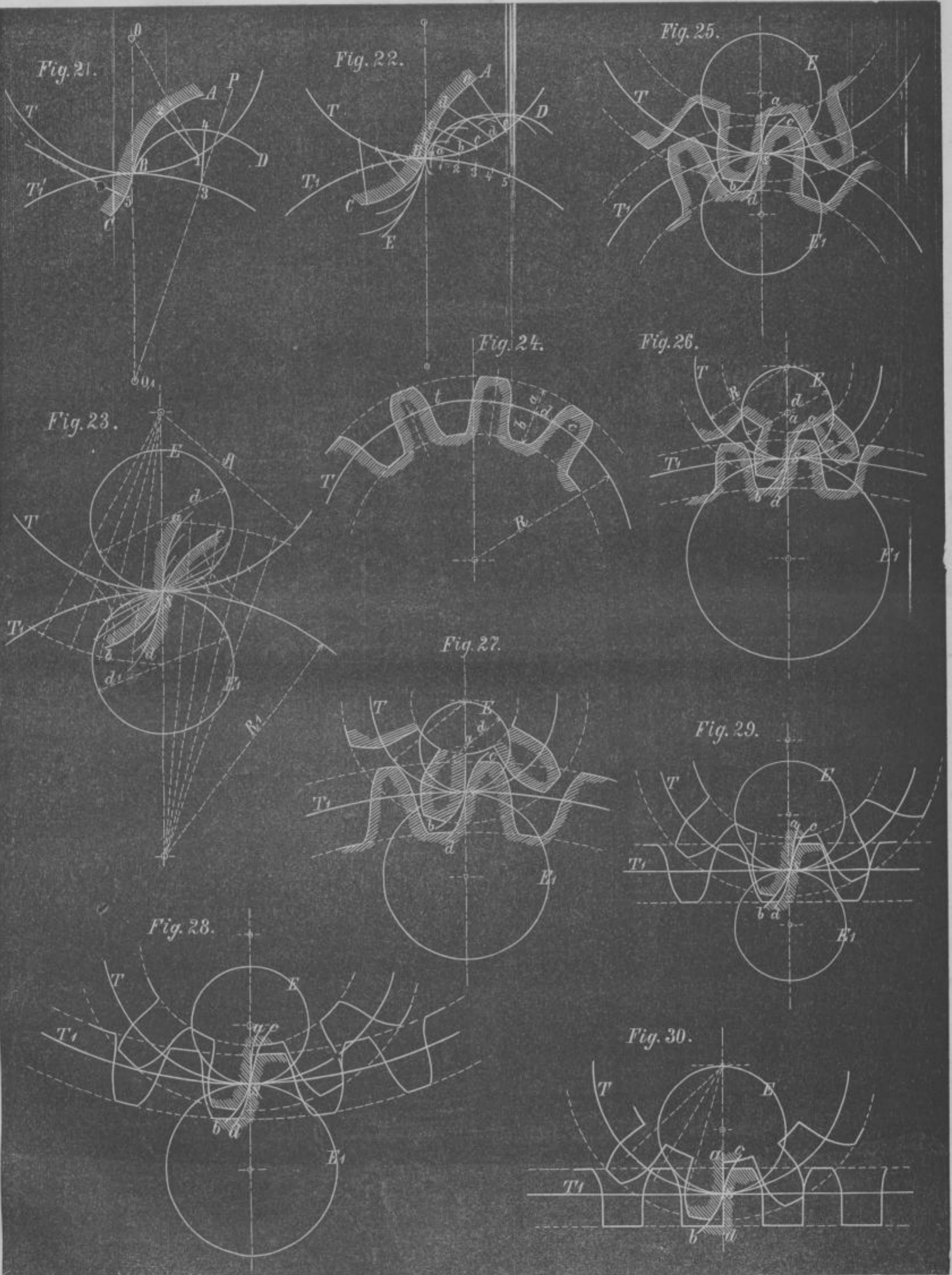
Ueber die Zahnconstruction der Zahnräder, von F. Stüßgen in Varep.
