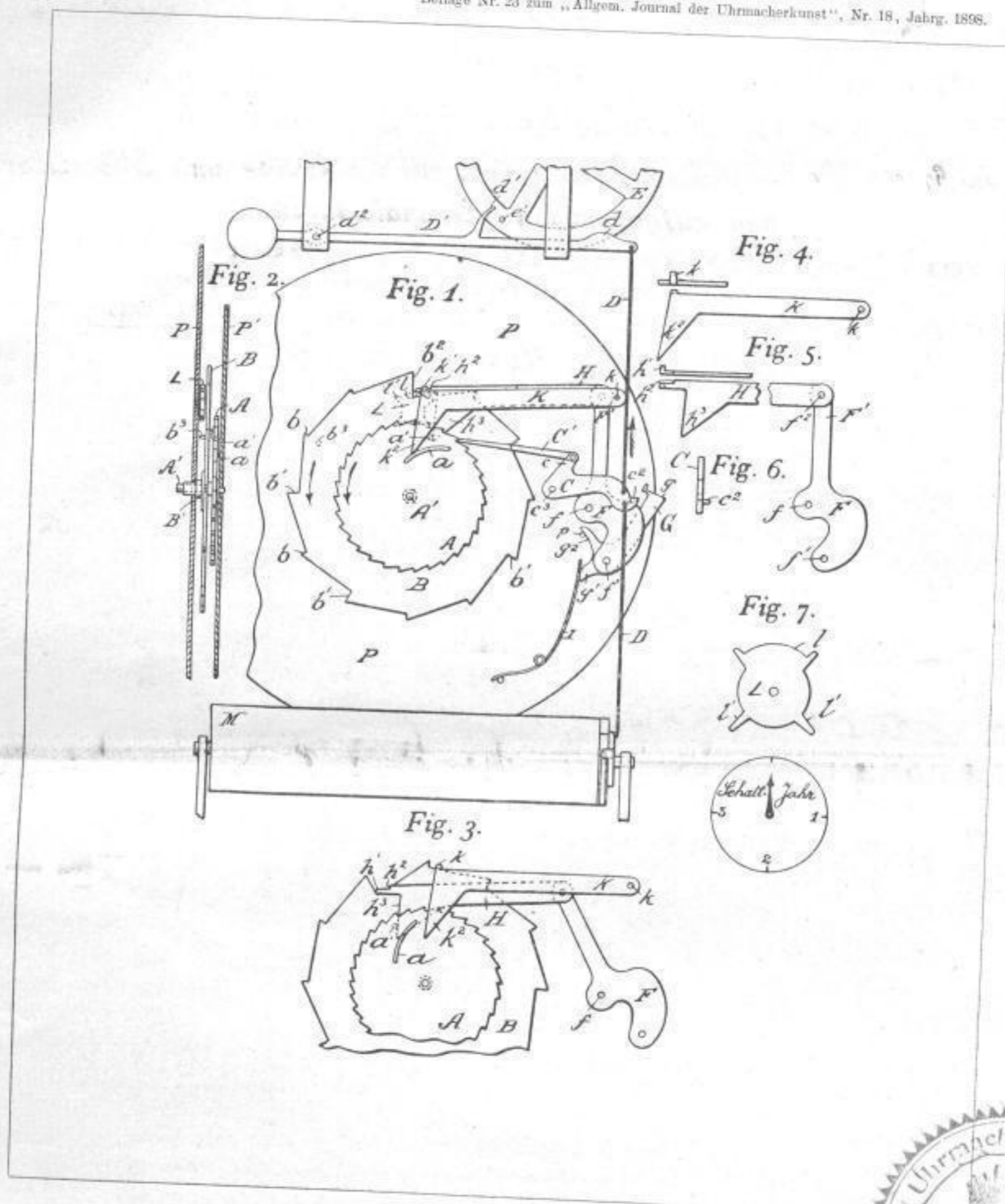
Zu dem Artikel: Vom Uhrwerk aus alle 24 Stunden geschaltete Kalenderuhr.
