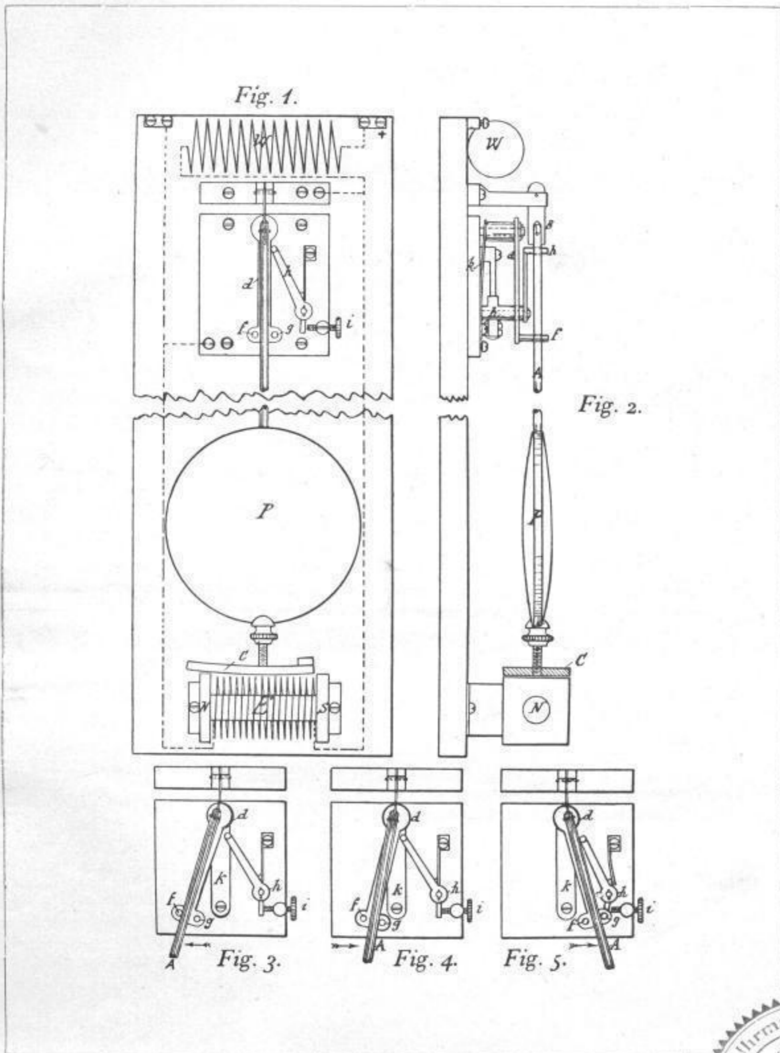
Verstellbare Stromschlussvorrichtung für elektrische Pendel, von Paul Rissler und Heinrich Bauer in Freudenstadt (Württemberg).
