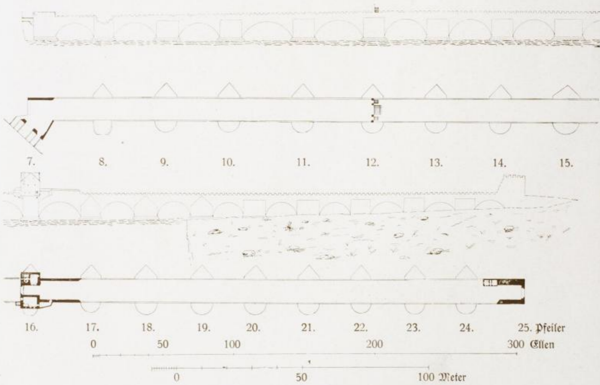
4. Plan der Brücke nach dem Zustand im Jahre 1559 (H. St. A.) (Wiedergegeben nach Gurlitt, Bau- und Kunstdenkmäler Sachsens.)
