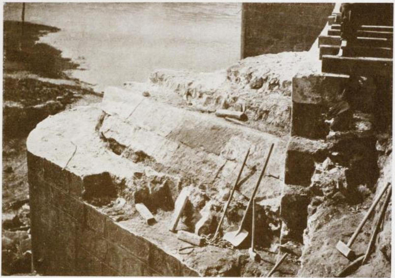
12. Freigelegter Vorkopf von Pfeiler 20.
