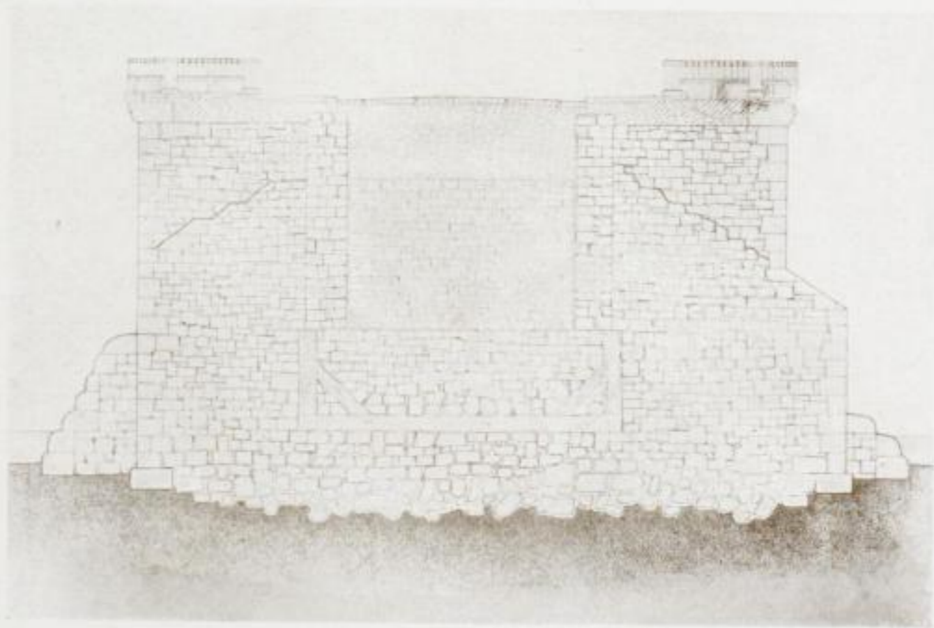
13. Querschnitt von Pfeiler 18. (Aufnahmezeichnung des Tiefbauamtes der Stadt Dresden.)
