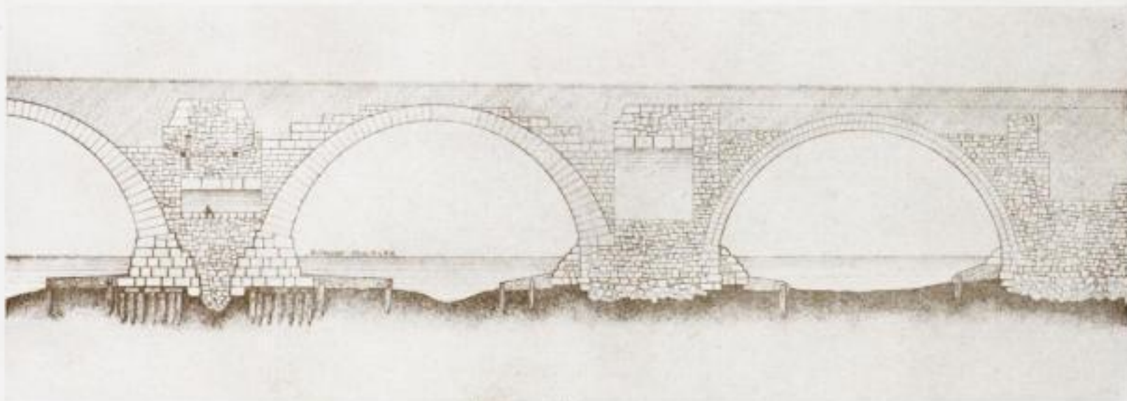
15. Längsschnitt von Pfeiler 15-17. (Aufnahmezeichnung des Tiefbauamtes der Stadt Dresden.)
