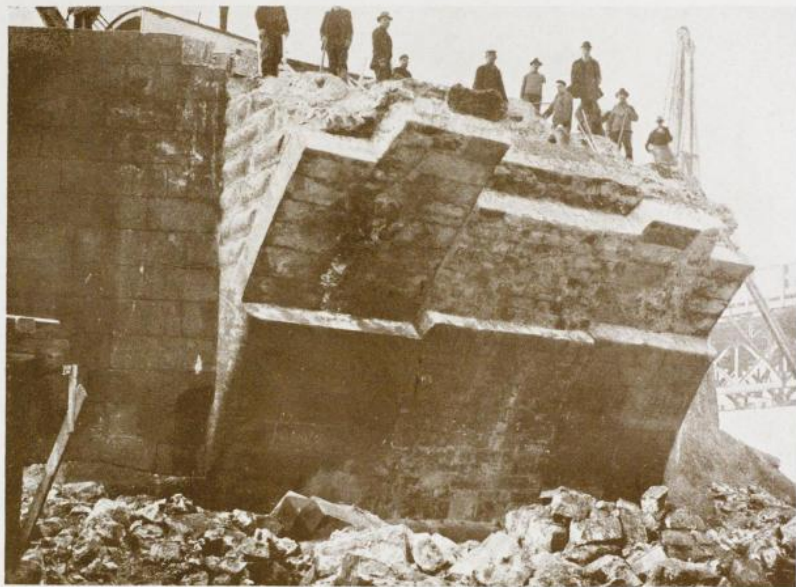
16. Abbruch des Bogens 16 (Zugbrückenbogen).
