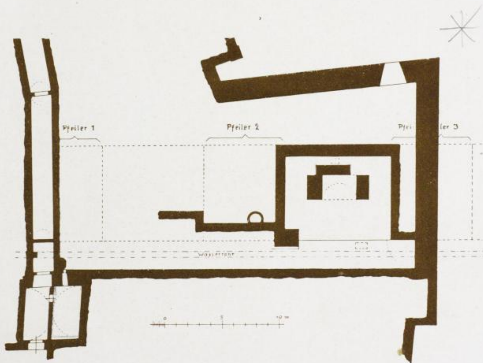
17. Kellergrundriß des Georgentores.
