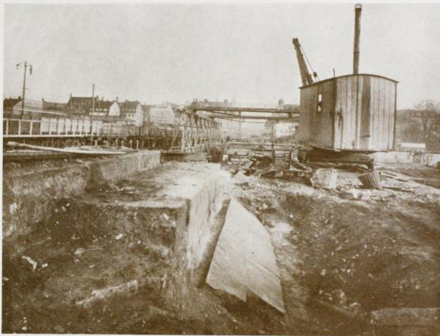
24. Schrägliegende Auflagerplatten der Zugbrücke bei Bogen 16.
