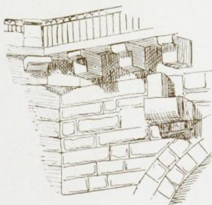
25. Einzelzeichnung vom Zugbrückenbogen. (Aus Gurlitt, Bau- und Kunstdenkmäler Sachsens.)
