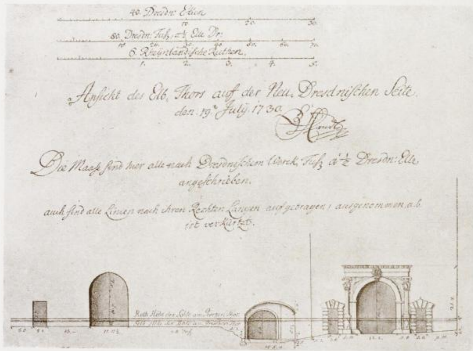
33. Ansicht des Elbtore 1730. (Hauptstaatsarchiv.)
