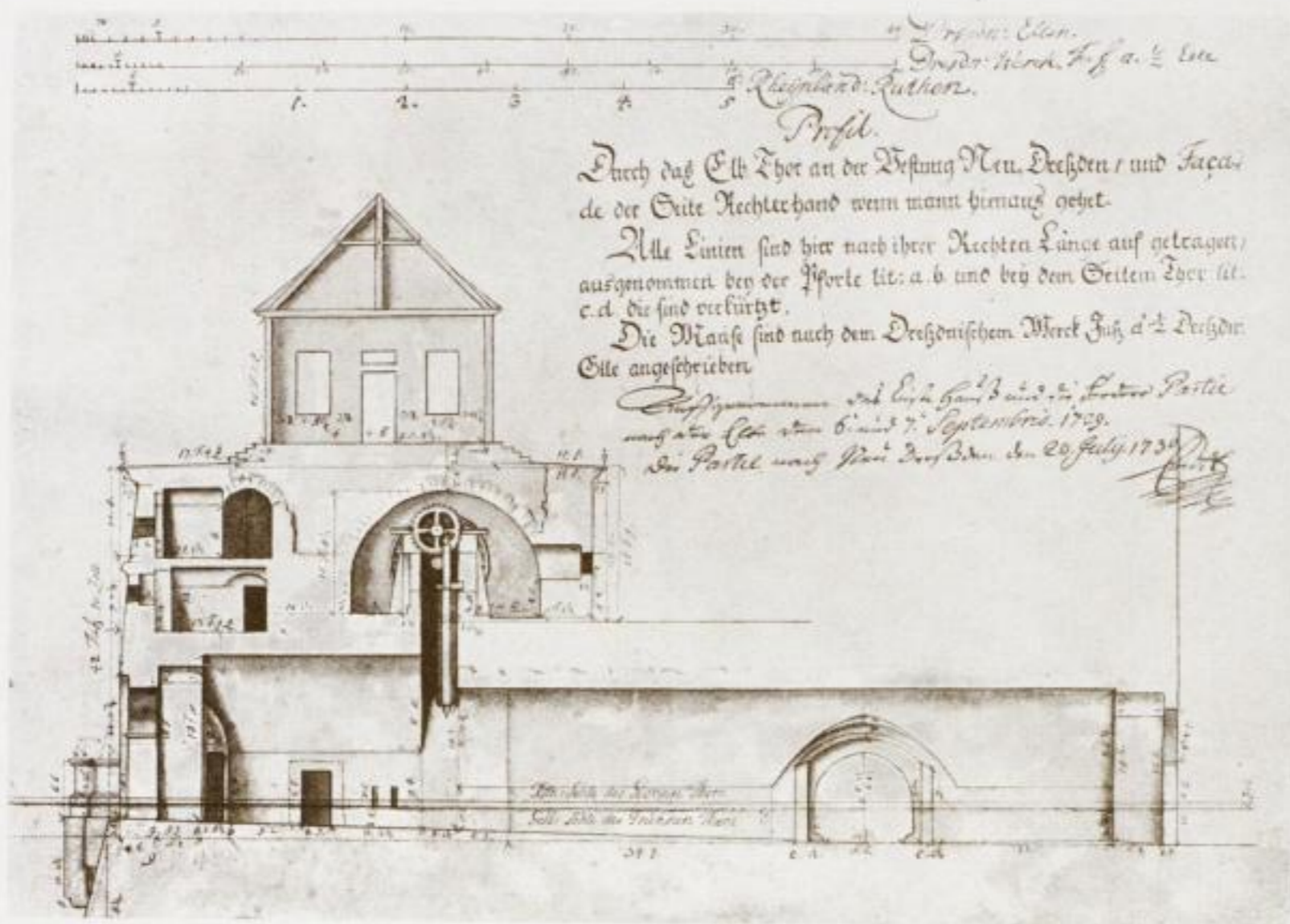
32. Schnitt durch das Elbtor. (Hauptstaatsarchiv.)
