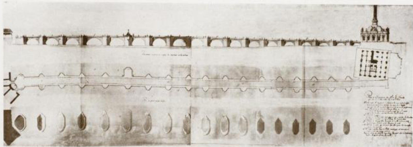
58. Gesamtbild der Brücke von 1728 mit dem Plan des Blockhauses. (Zuobergabe eines Planes im Denkmalsarchiv.)
