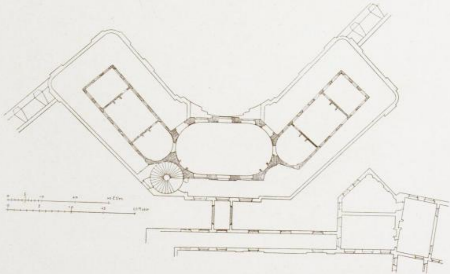
60. Grundriß vom Obergeschoß des Elbtors nach dem Entwurf von Longuelune. 1728. (Plan im Oberhofmarschallamt.)
