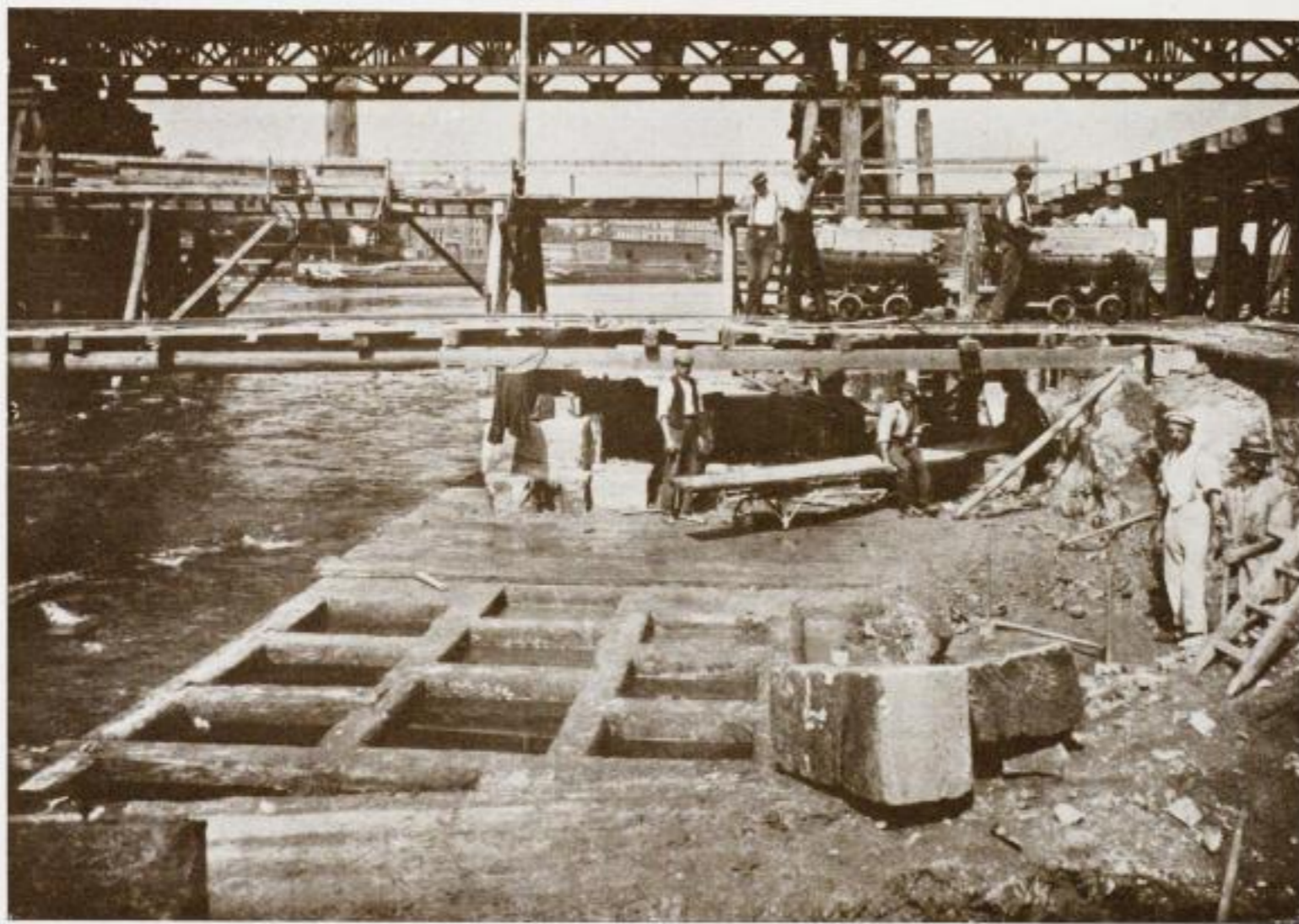
80. Aufgedeckter Koff des Pfeilers 15.
