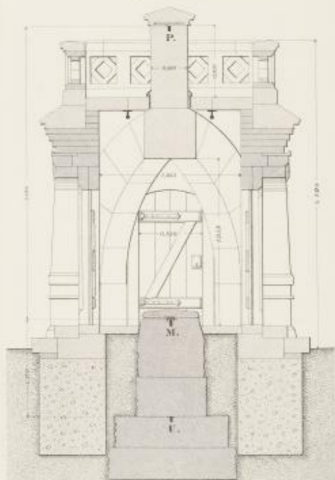
Querschnitt.
