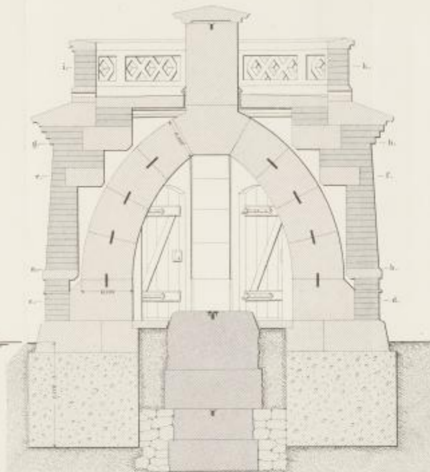
Diagonalschnitt.
