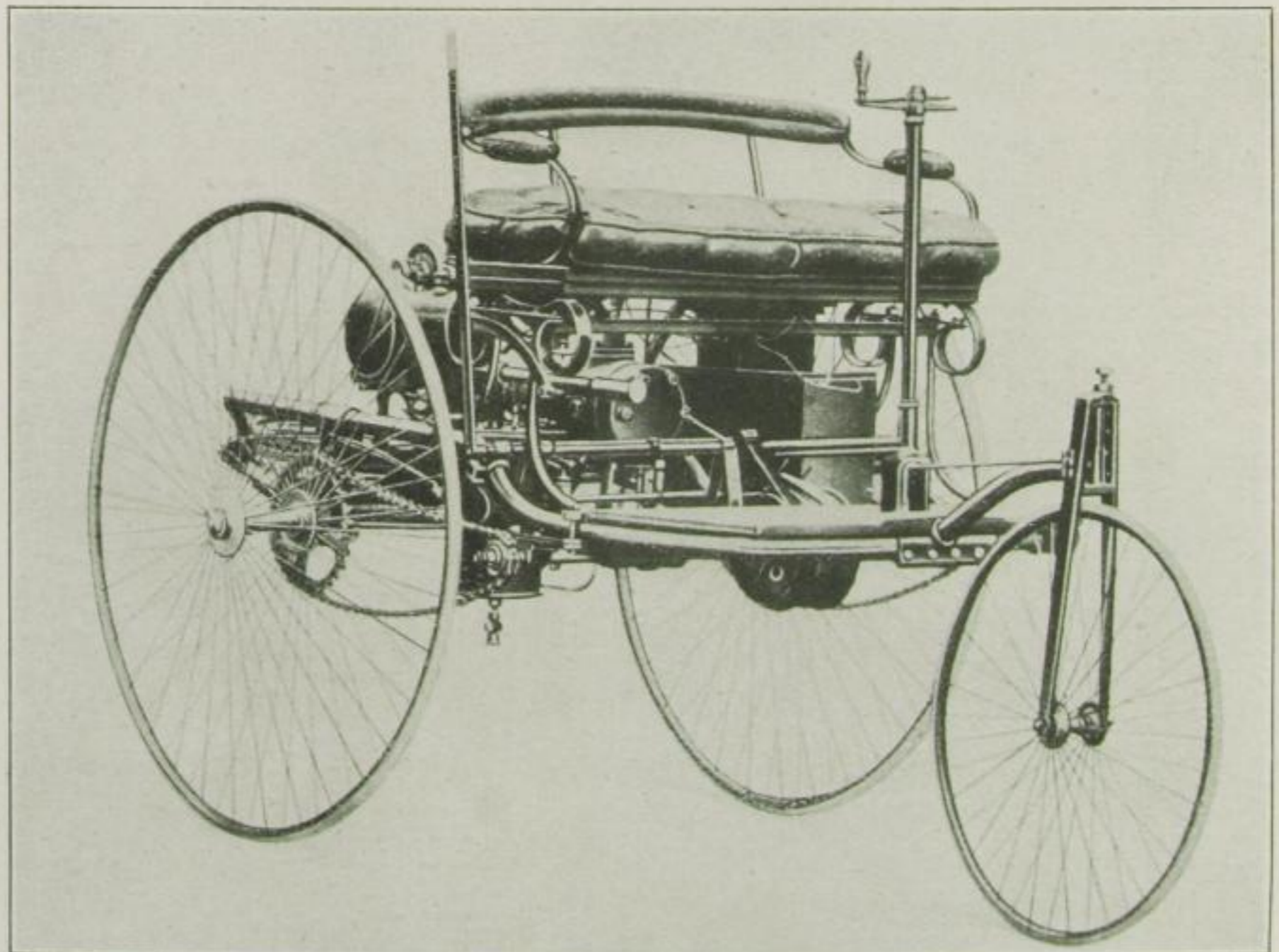
Ältestes Automobil aus dem Jahre 1886 von Carl Benz gebaut. Leistung \frac{1}{4} PS. Jetzt: Deutsches Museum, München
