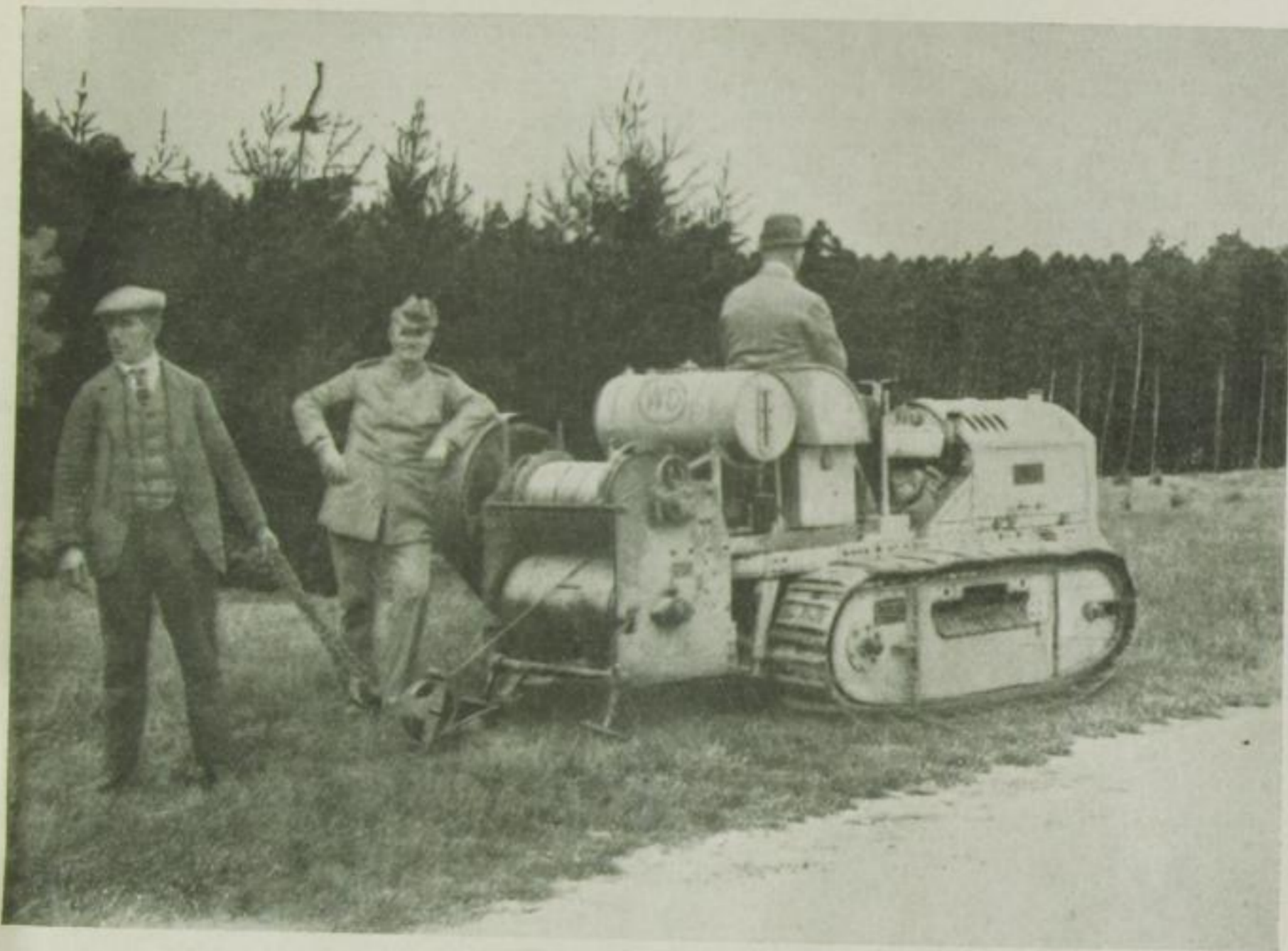
WD-Kleinschlepper mit anmontierter Rückenwinde bei der Waldarbeit
