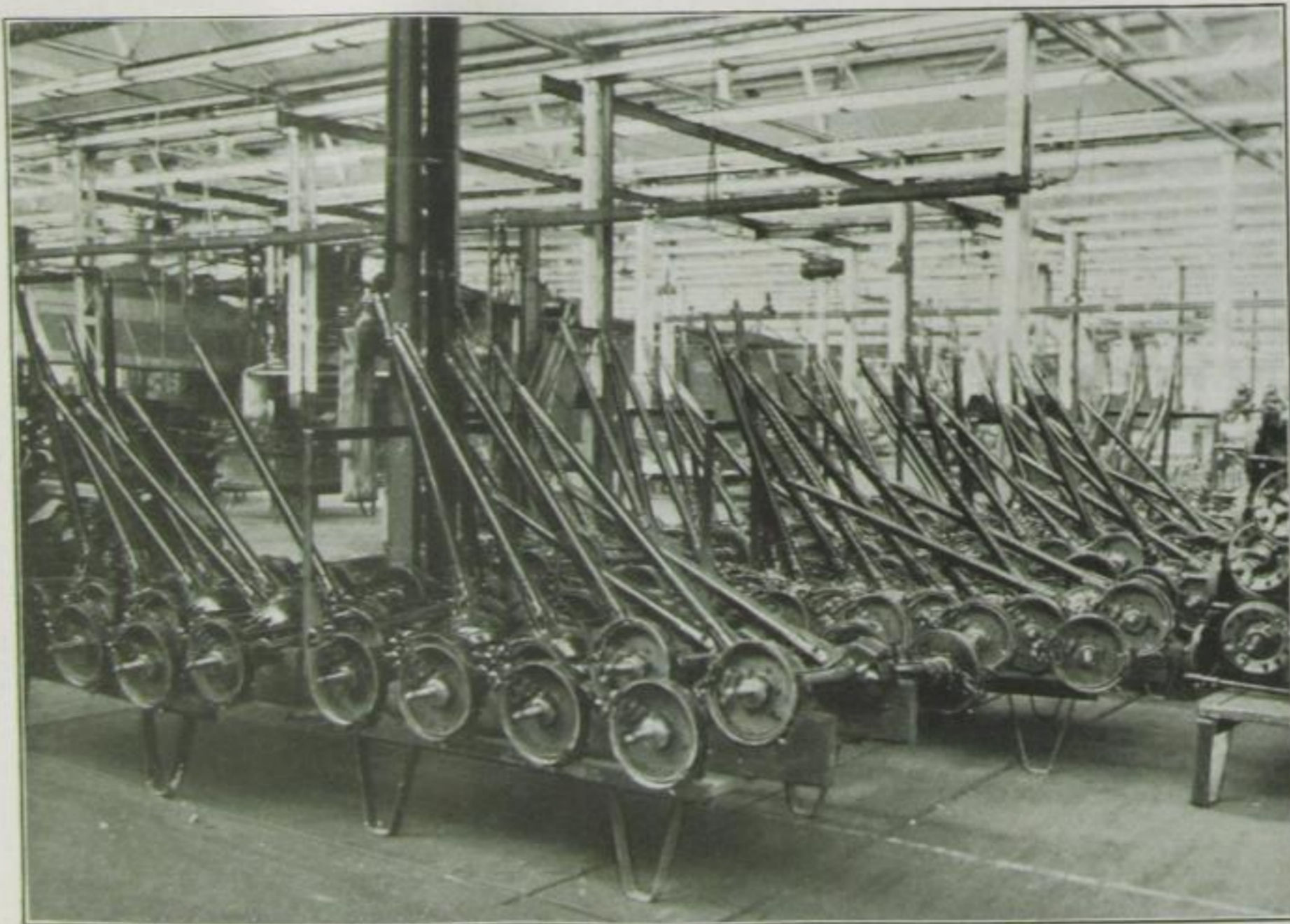
2. Fertige Hinterradachsen
