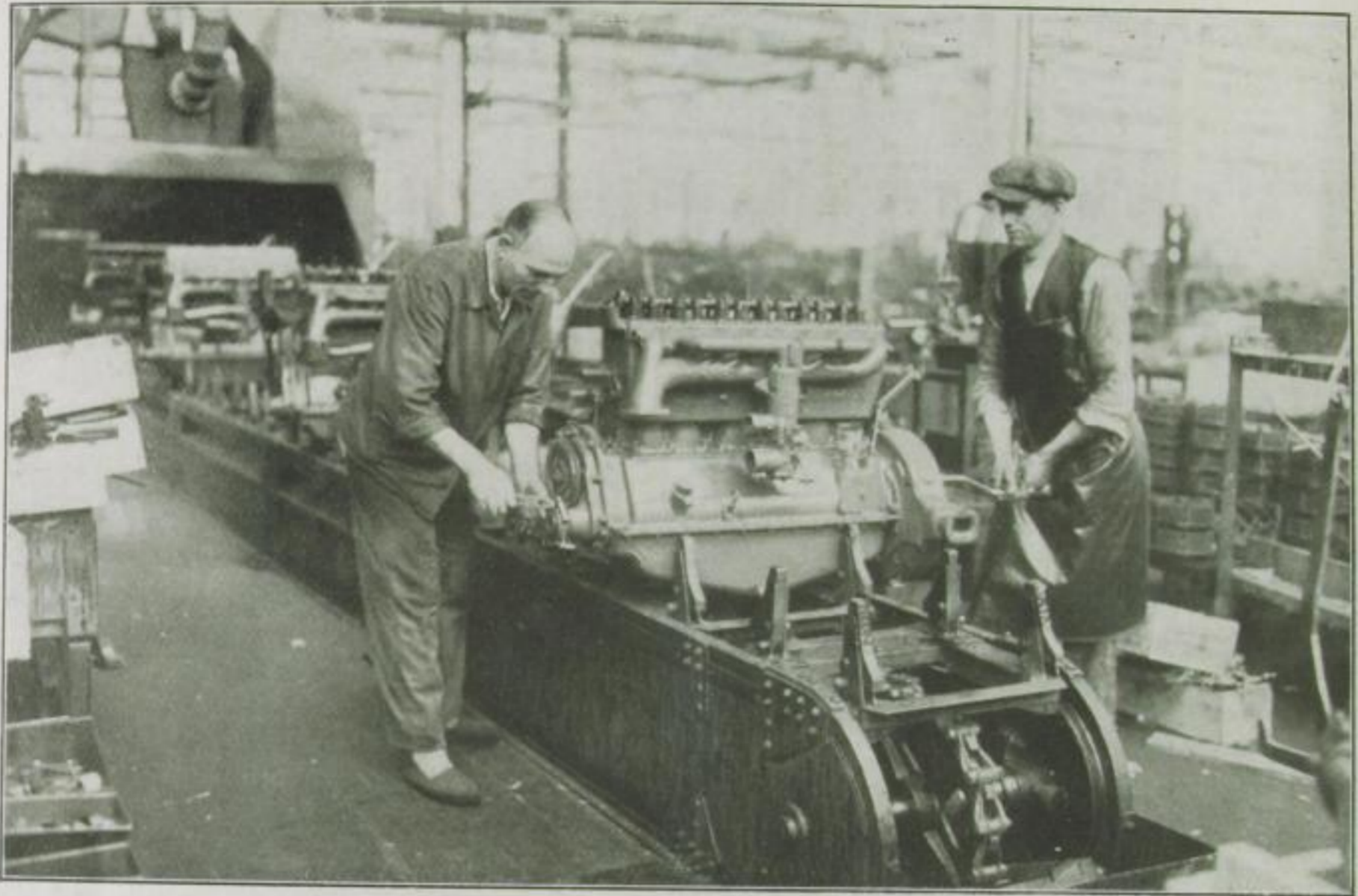
3. Vorbereitungen zum Einsetzen der Motoren
