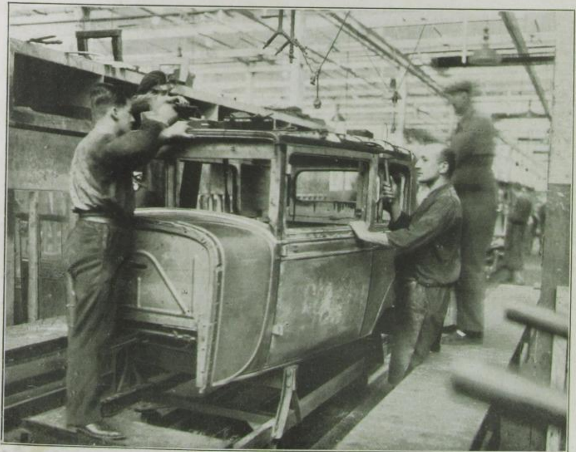
4. Anbringung von Türen und Fenstern
