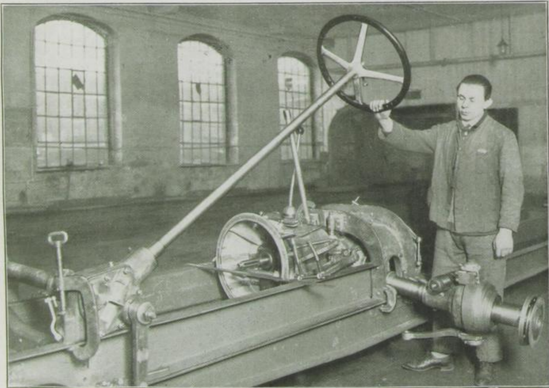
Vorderantrieb und Steuerung des neuen Rumpler-Vorderantrieblastwagens
