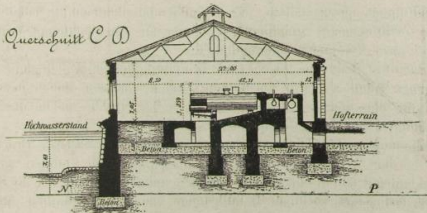
Fig. 259—262. Hauptwasserwerk der Stadt Dresden. (Wasserhebungsanlage).
